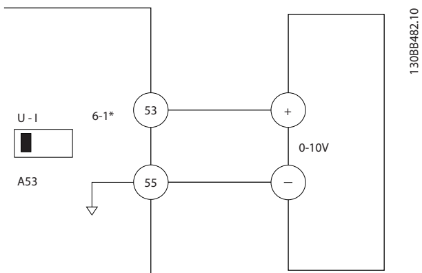
圖 5.1 提供 0-10V 控制信號之外部裝置的配線範例 (左為變頻器，右為外部裝置)
