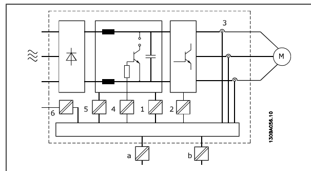
Galvanisk adskillelse
