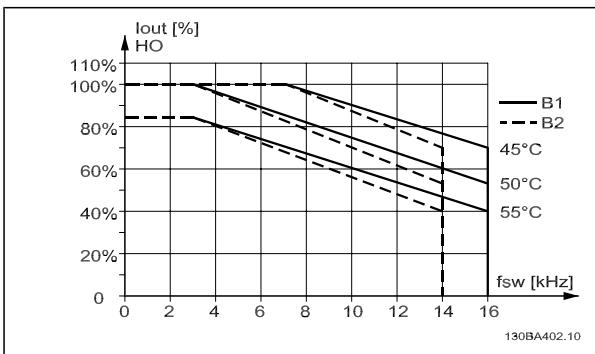
Derating af I_{out} for anden T_{OMG, MAKS} for kapsling B med 60 PWM i høj momenttilstand (160 % overmoment)
