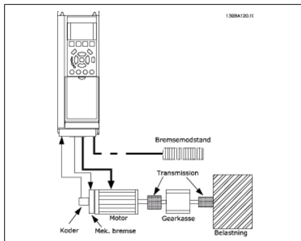
Grundlæggende opsætning for FC 302 ved hastighedsstyring med lukket sløjfe
