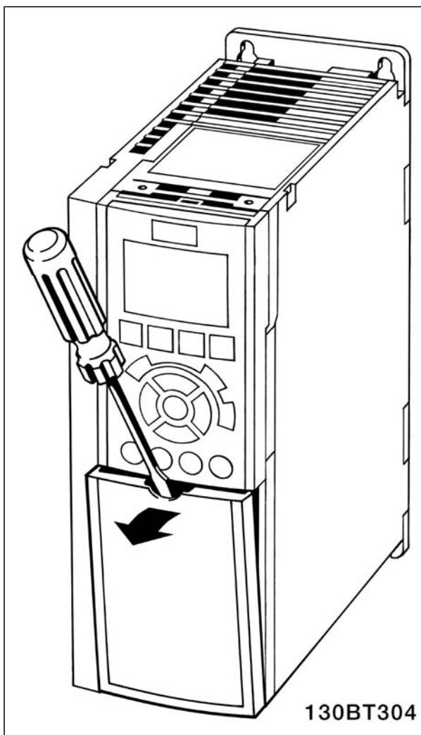
A1-, A2- og A3-kapslinger
