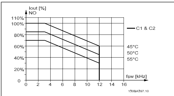
Derating af I_{out} for anden T_{OMG, MAKS} for kapsling C med 60 PWM i normal momenttilstand (110 % overmoment)
