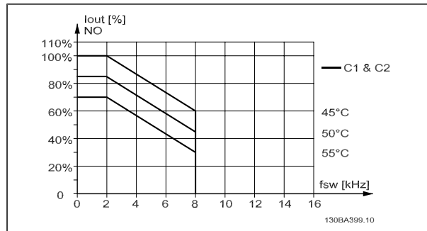
Derating af I_{out} for anden T_{OMG, MAKS} for kapsling C med SFAVM i normal momenttilstand (110 % overmoment)
