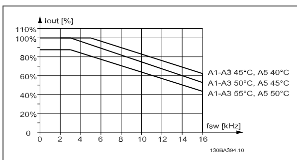
Derating af I_{out} for anden T_{OMG,MAKS} for kapsling A med 60 PWM og maks. 10 m motorkabel
