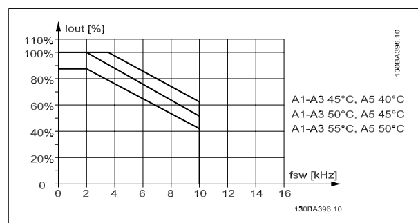
Derating af I_{out} for anden T_{OMG,MAKS} for kapsling A med SFAVM og maks. 10 m motorkabel
