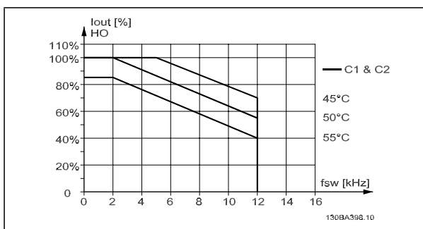
Derating af I_{out} for anden T_{OMG, MAKS} for kapsling C med 60 PWM i høj momenttilstand (160 % overmoment)
