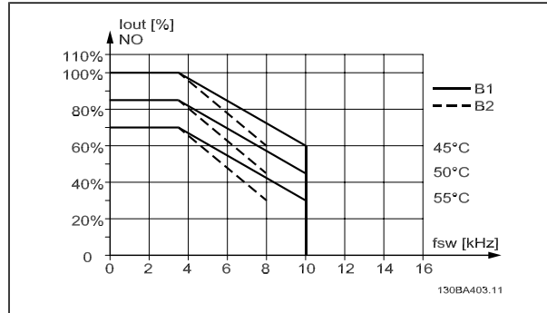
Derating af I_{out} for anden T_{OMG, MAKS} for kapsling B med SFAVM i normal momenttilstand (110 % overmoment)
