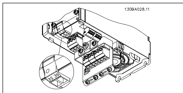
Tilslutning til 24 V backup-forsyning på rammestørrelser A2 og A3.
