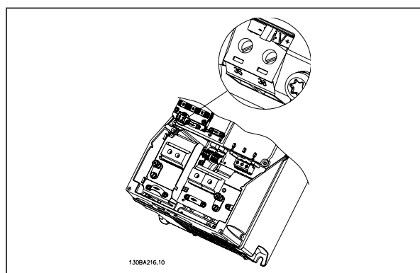
Tilslutning til 24 V backup-forsyning på rammestørrelser A2 og A3.
