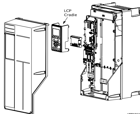
Rammestørrelse A5, B1, B2, C1 og C2
