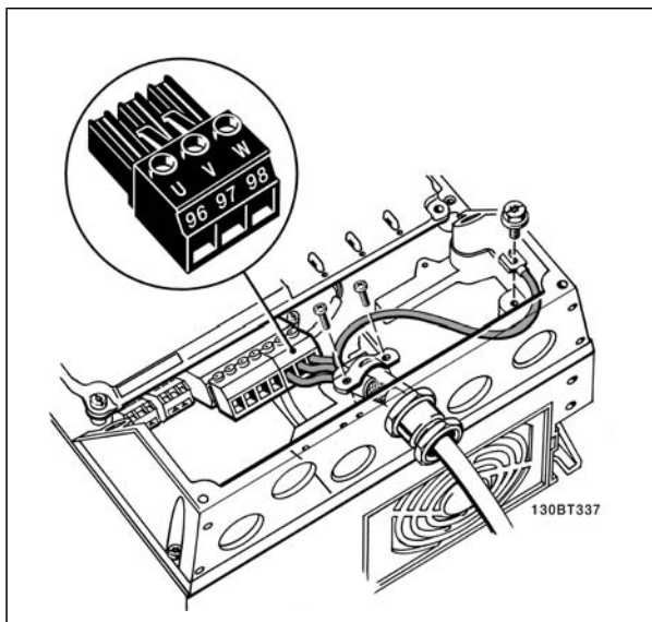
Motortilslutning til A5-kapsling (IP55/66/NEMA Type 12)
