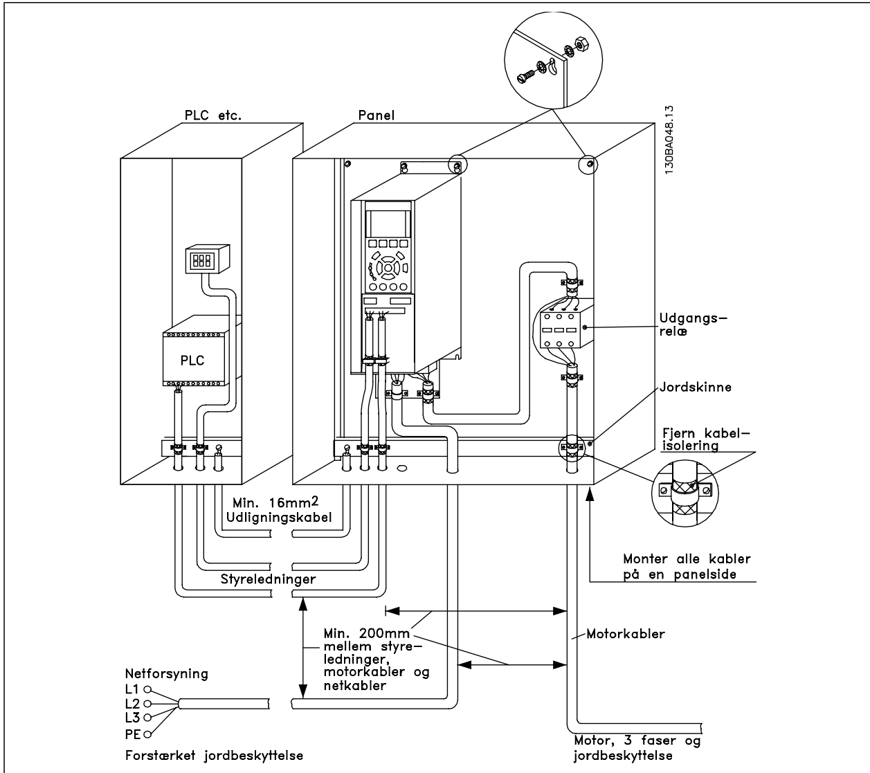
EMC-korrekt elektrisk installation af en IP 20 -frekvensomformer.
