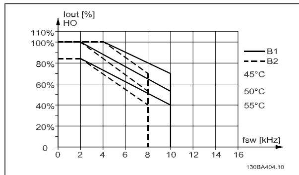
Derating af I_{out} for anden T_{OMG, MAKS} for kapsling B med SFAVM i høj momenttilstand (160 % overmoment)
