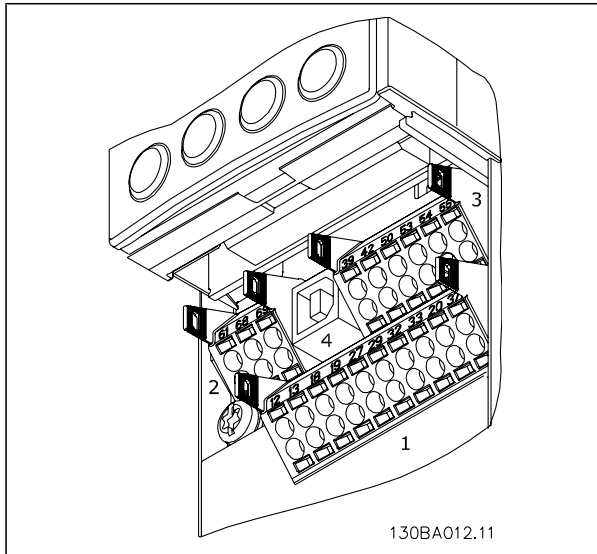
Styreklemmer (alle kapslinger)
