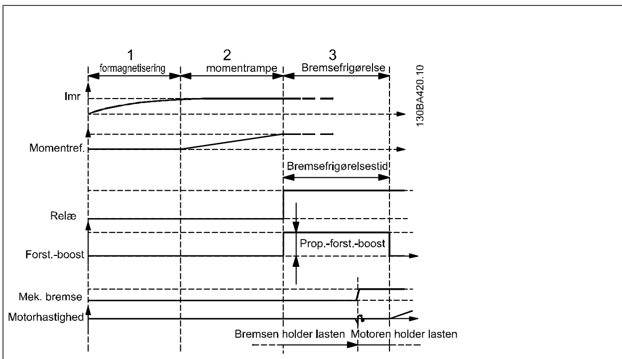
Bremsefrigørelsessekvens for hæve/sænke-mekanisk bremsestyring
