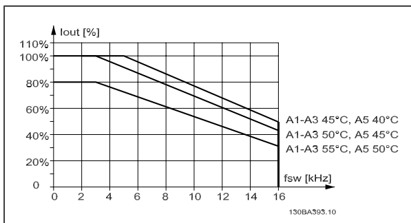
Derating af I_{out} for anden T_{OMG,MAKS} for kapsling A med 60 PWM
