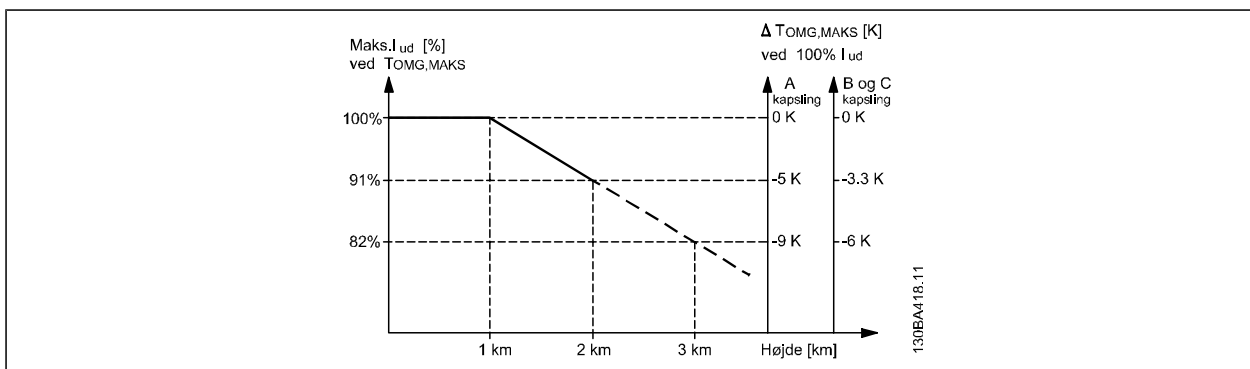
Derating af udgangsstrøm kontra højde ved T_{OMG, MAKS} . Ved højder over 2 km skal Danfoss Drives kontaktes vedr. PELV.
