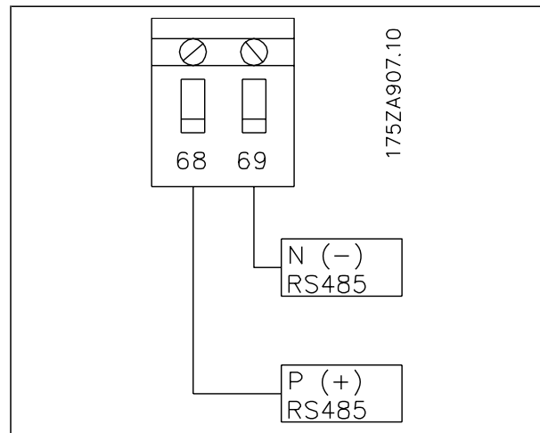
Netværksklemmeforbindelse
