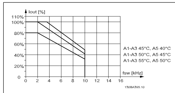
Derating af I_{out} for anden T_{OMG,MAKS} for kapsling A med SFAVM
