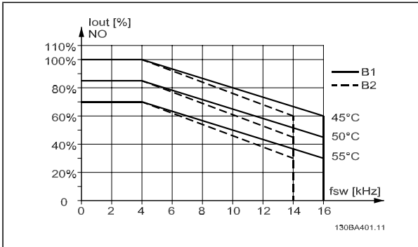
Derating af I_{out} for anden T_{OMG, MAKS} for kapsling B med 60 PWM i normal momenttilstand (110 % overmoment)
