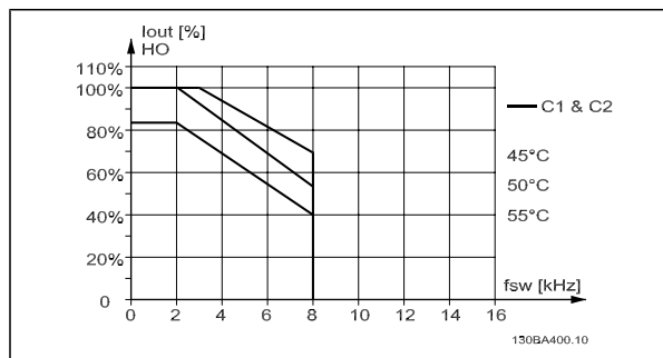
Derating af I_{out} for anden T_{OMG, MAKS} for kapsling C med SFAVM i høj momenttilstand (160 % overmoment)
