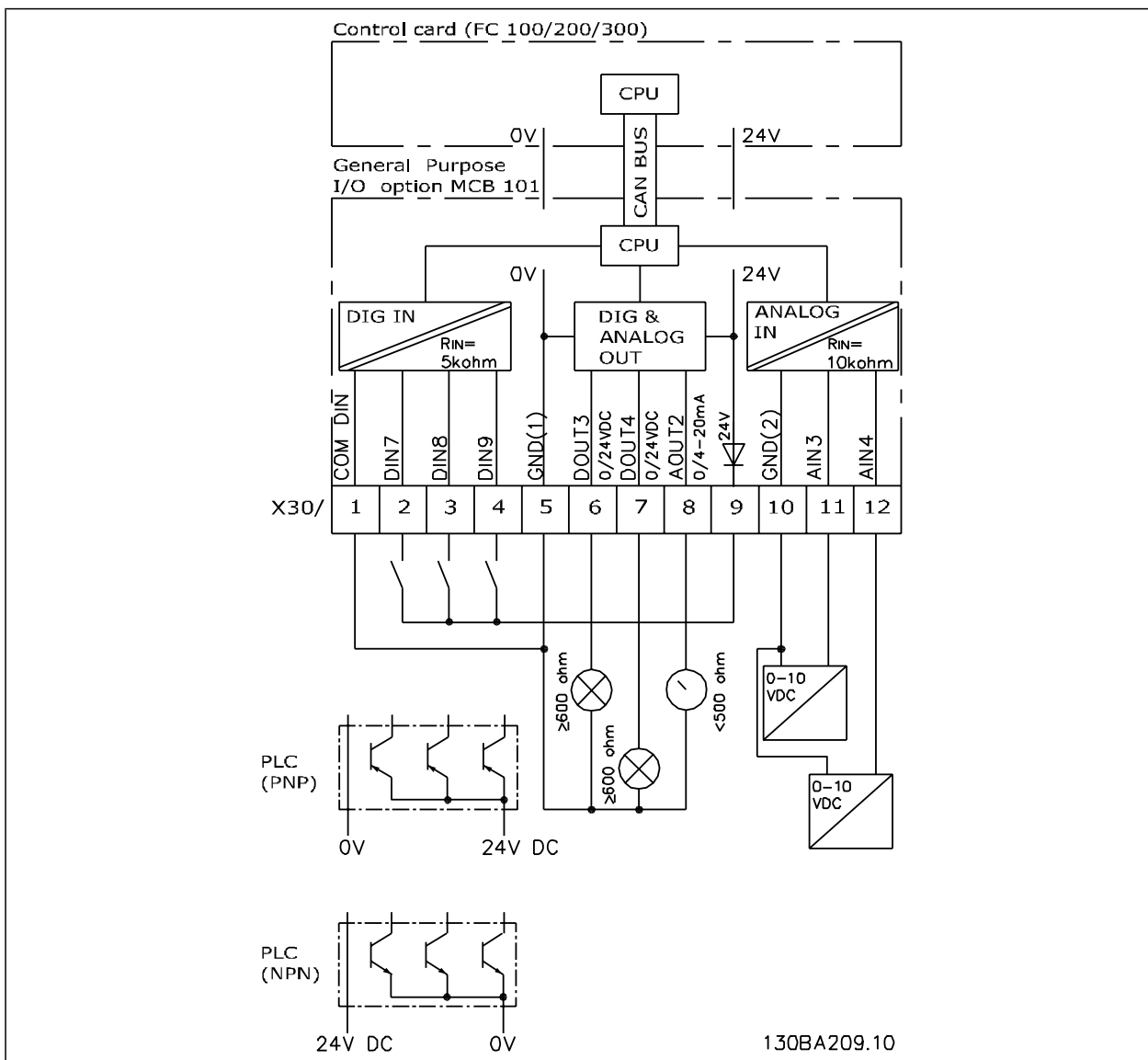
Principdiagram
