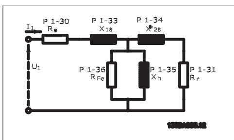
Abbildung 2.1: Ersatzschaltbild eines Asynchronmotors
