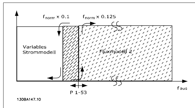
Abbildung 2.3: Par. 1-00 = [0] Ohne Rückführung Par. 1-01 = [2] Fluxvektor ohne Geber
