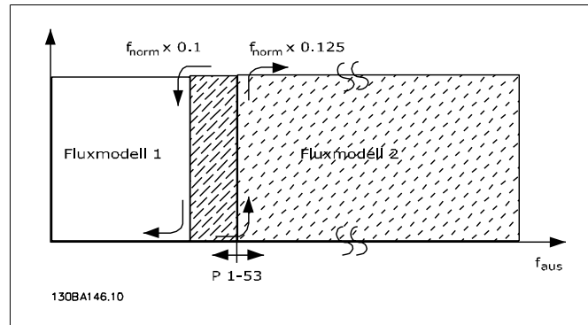
Abbildung 2.2: Funktion bei Fluxvektor mit Geber Par. 1-01 = [3]
