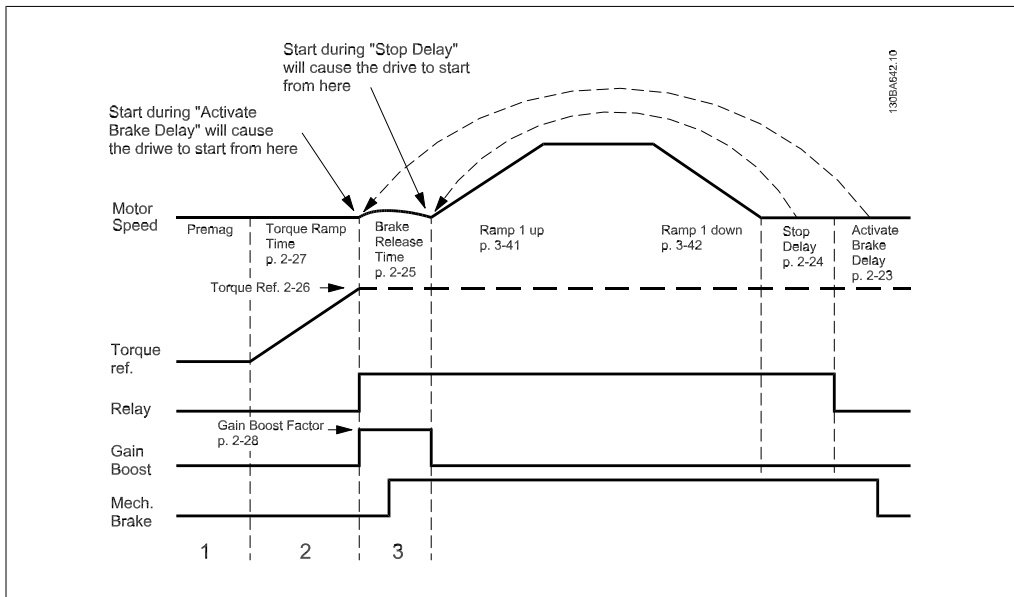
Abbildung 2.4: Sequenz zum Lüften der Bremse bei mechanischer Bremsansteuerung für Vertikalförder- und Hubanwendungen
