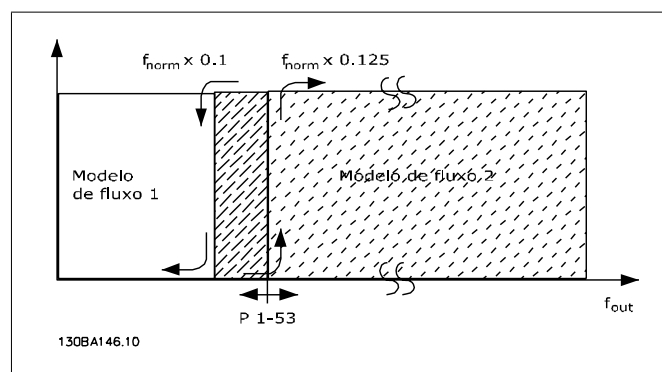
Ilustração 2.2: Par. 1-00 = [1] Malha fech. veloc. ou [2] Torque e par. 1-01 = [3] Flux c/ feedb. motor
