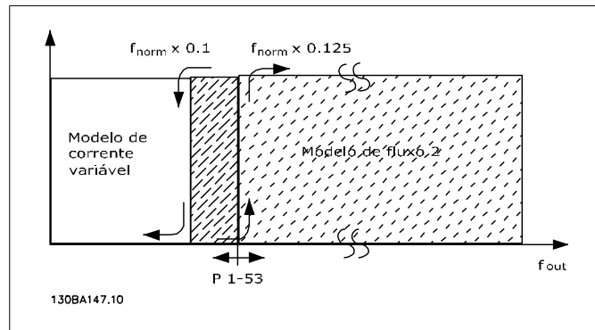
Ilustração 2.3: o par. 1-00 = [0] Malha aberta veloc. Par. 1-01 = [2] Flux Sensorless
