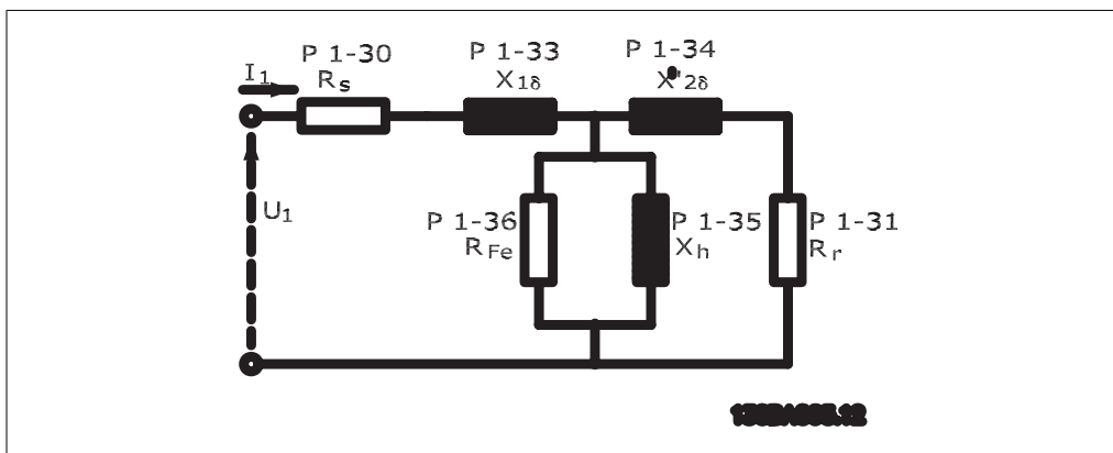
Ilustração 2.1: Diagrama equivalente de motor referente a um motor assíncrono
