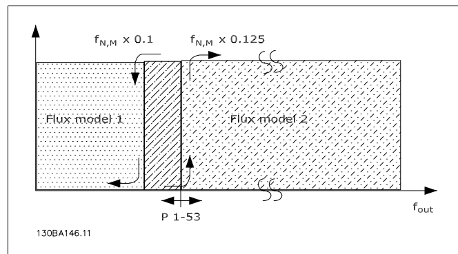
图 2.2: 参数 1-00 = [1] 闭环速度或 [2] 转矩，参数 1-01 = [3] 磁通矢量带电动机反馈
