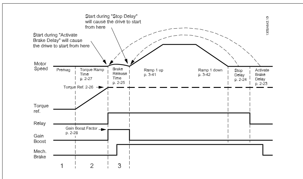
图 2.4: 起重机械制动控制的抱闸释放过程
