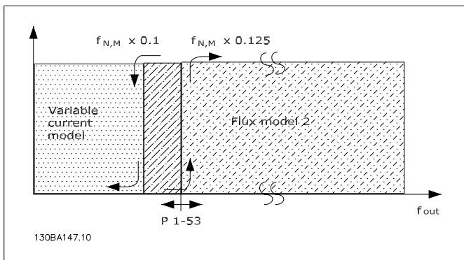
图 2.3: 参数 1-00 = [0] 开环速度 参数 1-01 = [2] 无传感器矢量
