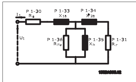
图 2.1: 异步电动机的电动机当量图
