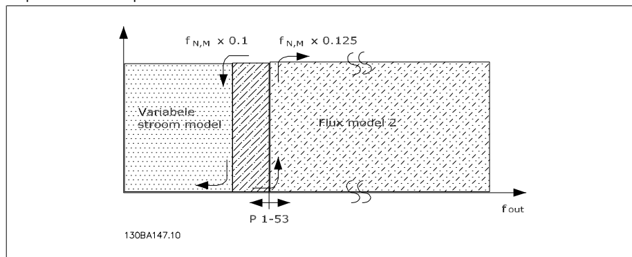
Afbeelding 2.3: Par. 1-00 = Snelheid open lus [0]
