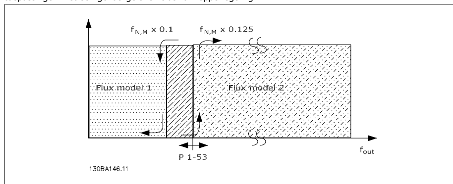
Afbeelding 2.2: Par. 1-00 = Snelheid gesl. lus [1] of Koppel [2] en par. 1-01 = Flux met enc.terugk. [3]
