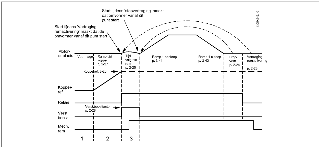
Afbeelding 2.4: Remvrijgaveprocedure voor mechanische rembesturing bij hijstoepassingen
