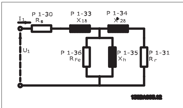
Afbeelding 2.1: Motorequivalentiediagram voor een asynchrone motor
