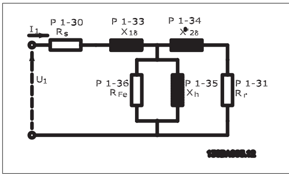
图 2.1: 异步电动机的电动机当量图
