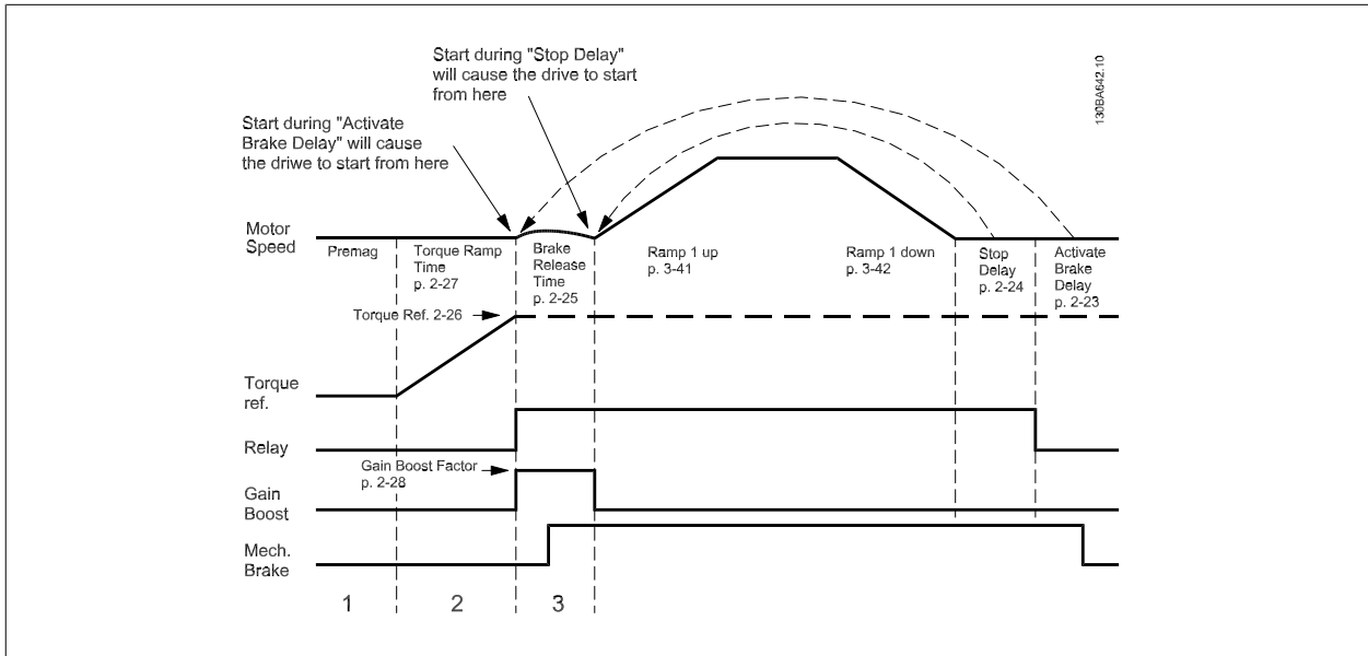
图 2.4: 起重机机械制动控制的抱闸释放过程
