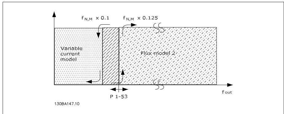
图 2.3: 参数 1-00 = [0] 开环速度 参数 1-01 = [2] 无传感器矢量
