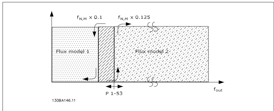
图 2.2: 参数 1-00 = [1] 闭环速度或 [2] 转矩, 参数 1-01 = [3] 磁通矢量带电动机反馈
