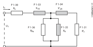
Illustration 3.1: Diagramme d'équivalence moteur pour un moteur asynchrone
