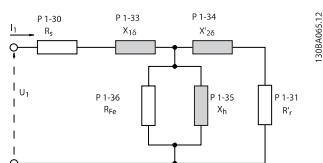
Рисунок 3.1: Эквивалентная схема асинхронного двигателя
