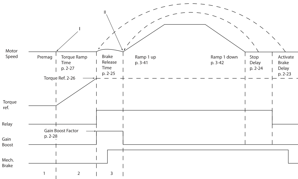
图 3.4: 起重机械制动控制的抱闸释放过程
