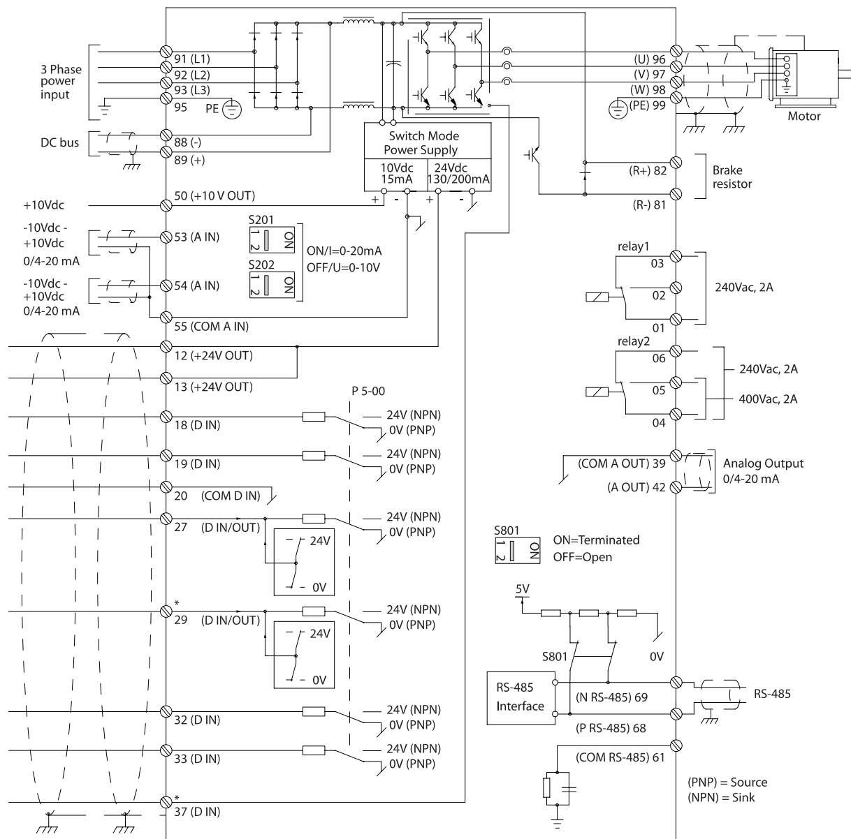
图 1.1: 图中显示了不带选件时的所有电气端子。
