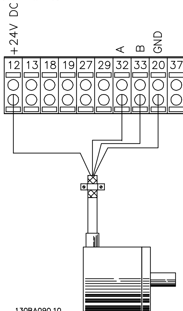
图 3.5: 24 V 增量编码器。电缆最大长度 5 m。
