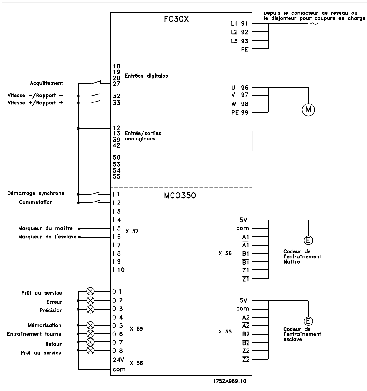
Schéma de câblage - régulation d'un convoyeur à bande
