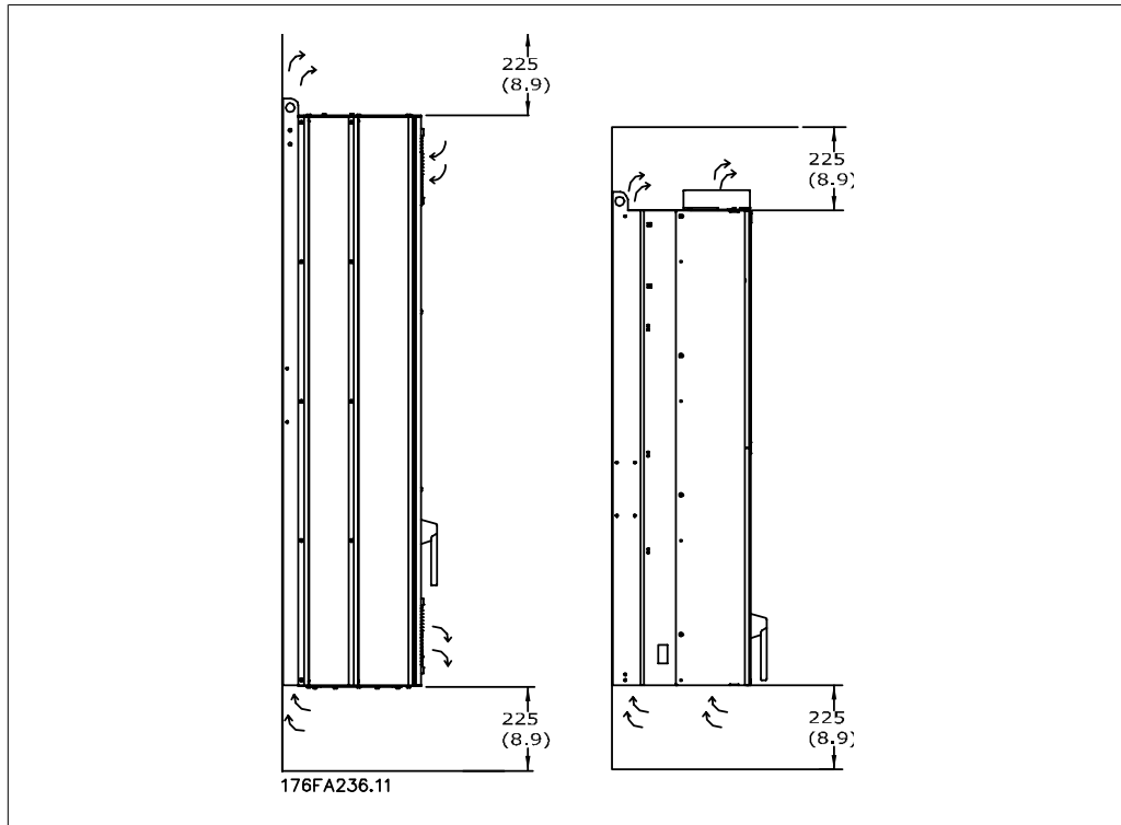
圖 3.6: 冷卻氣流的方向與必要的空間
