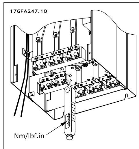
圖 3.79: 務必使用扭力扳手將螺栓扭緊。
