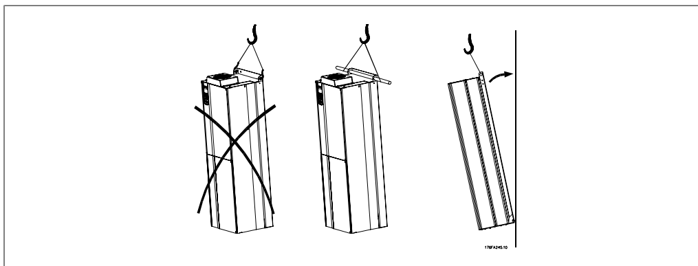
圖 3.21: 將變頻器固定在牆上的吊掛方式
