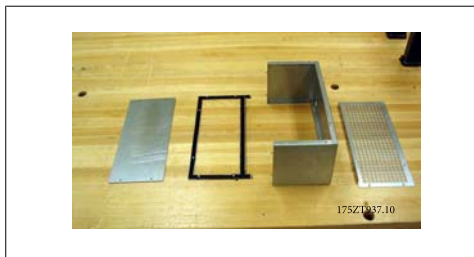
圖 3.37: 上方導管組零件
