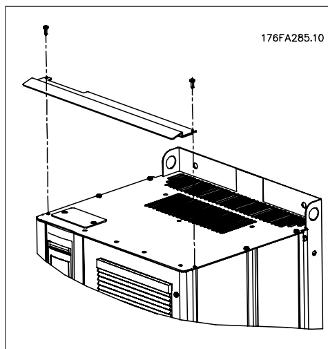
圖 3.28: 滴漏防護安裝。
