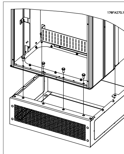
圖 3.24: 將變頻器安裝至基座
