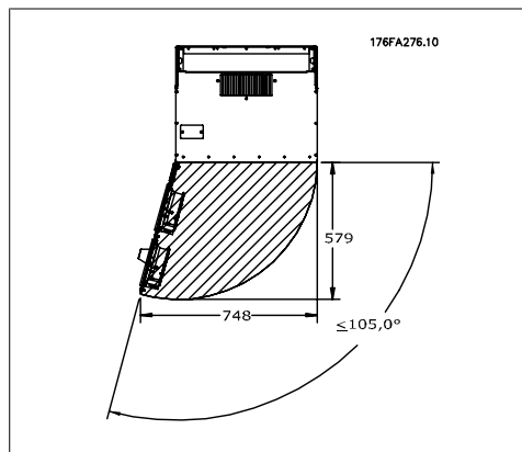
圖 3.5: IP21/IP54 外殼類型為 E1 的前方空間。
