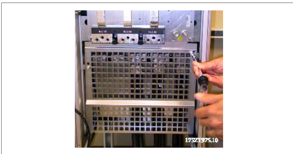
圖 3.81：EMC 防護裝置的安裝。
