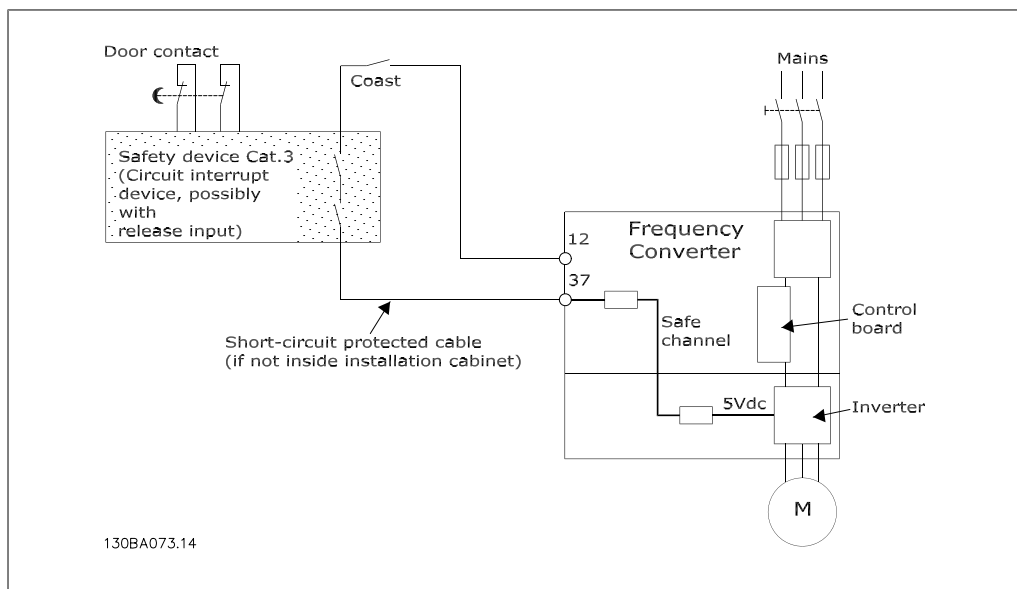
圖 2.2: 下圖顯示了一個符合安全類別 3 (EN 954-1) 的停止類別 0 (EN 60204-1) 的安裝所需的基本配置。
