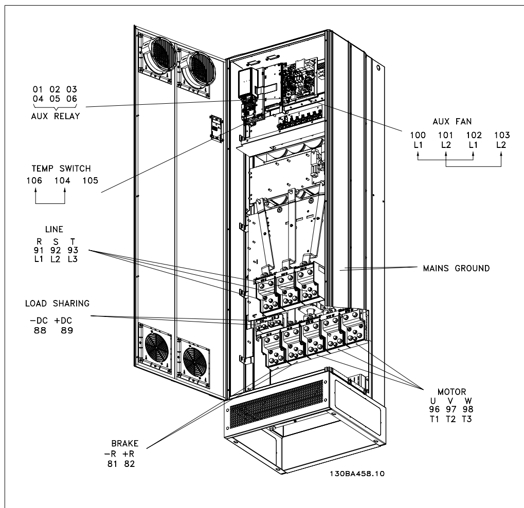
圖 3.78: 精巧型 IP 21 (NEMA 1) 與 IP 54 (NEMA 12), 外殼 E1
