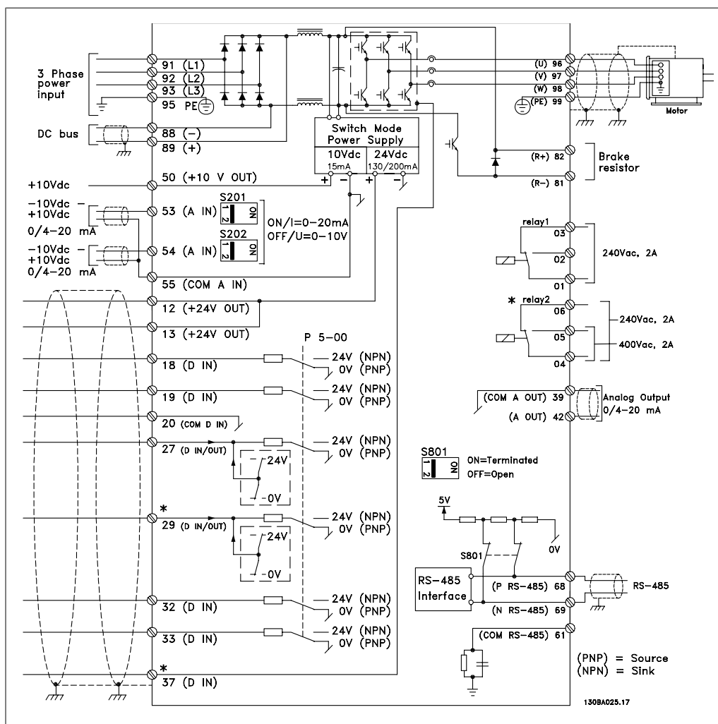
圖 3.82: 顯示所有不含選項電氣端子的圖表。
