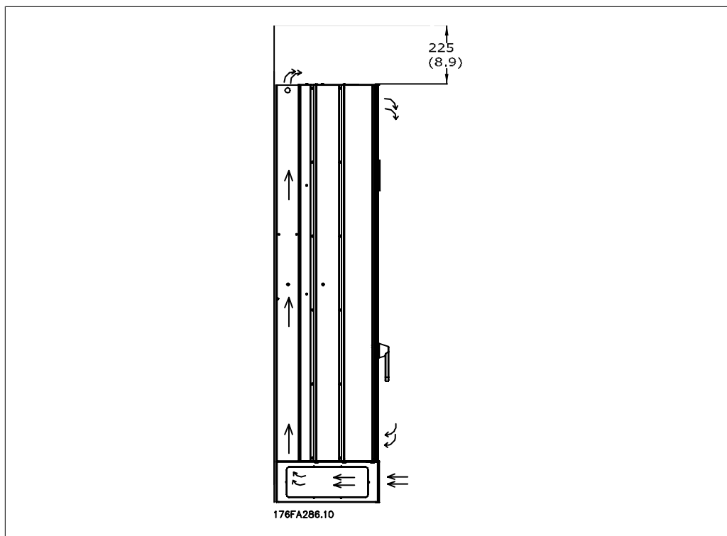
圖 3.7: 冷卻氣流的方向與必要的空間 - 外殼 IP21/54, E1
