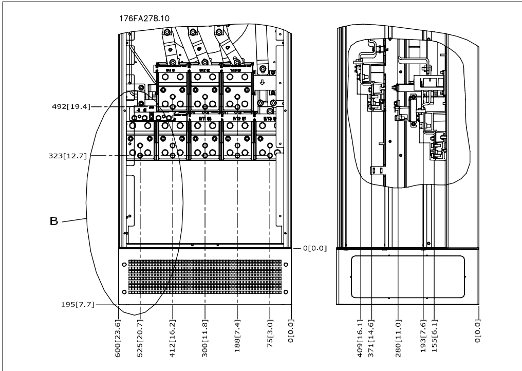
圖 3.10: IP21 (NEMA 類型 1) 與 IP54 (NEMA 類型 12) 外殼電源連接位置
