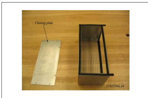
圖 3.45: 裝有墊片的上方導管
