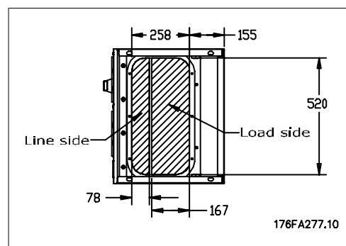
圖 3.26: 從變頻器底部所看到的電纜線入口 - 外殼 E1。
