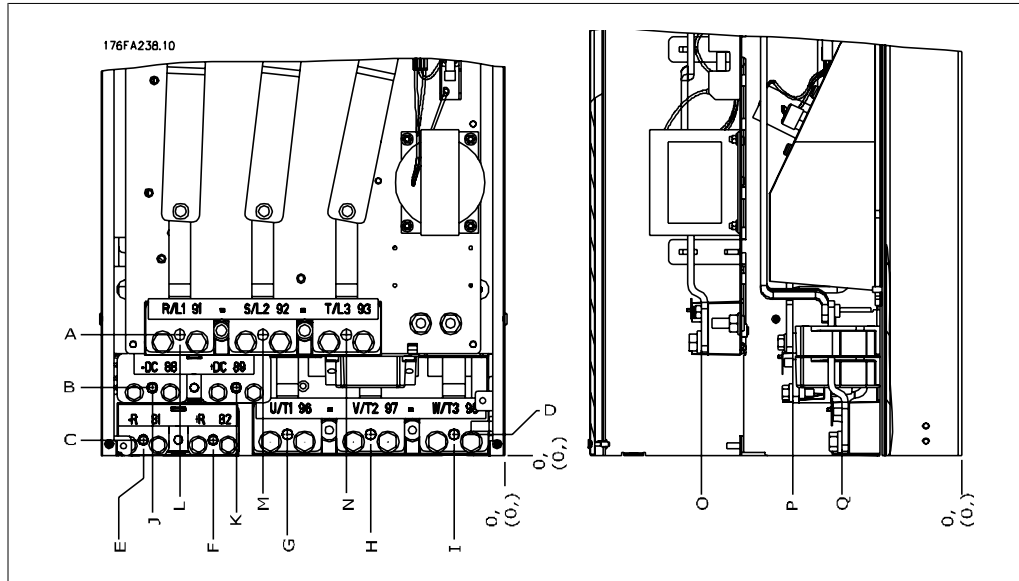
圖 3.8: 電源連接的位置
