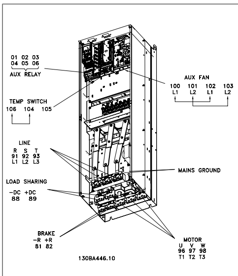
圖 3.70: 精巧型 IP 00 (底架), 外殼 D3
