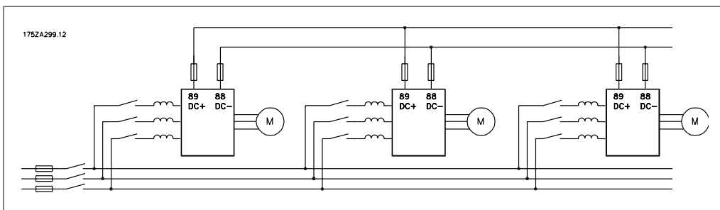
圖 3.80：負載共償連接。
