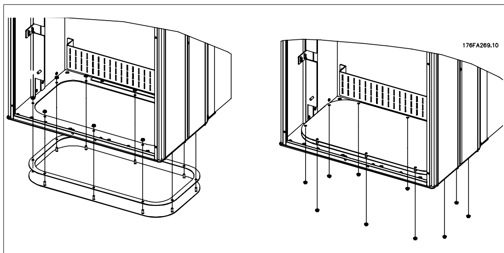
圖 3.27: 底板的安裝，E1 外殼。
