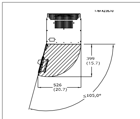
圖 3.4: IP21/IP54 外殼類型為 D1 與 D2 的前方空間。
