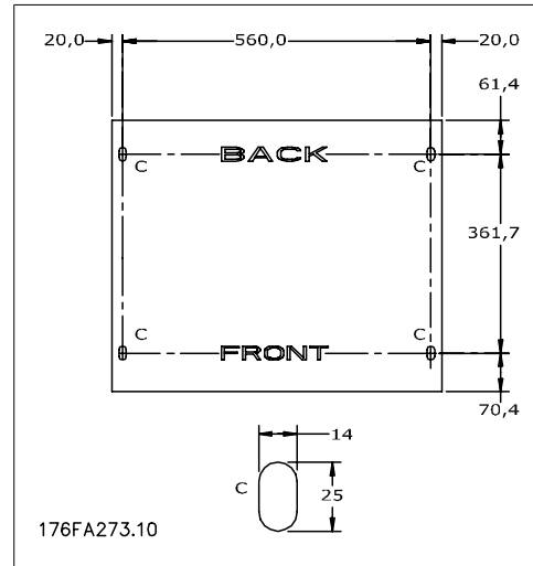
圖 3.23: 鑽孔工具是用來鑽地板上的固定孔。
