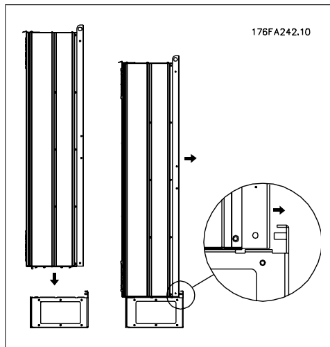
圖 3.64：將變頻器裝上基座。
