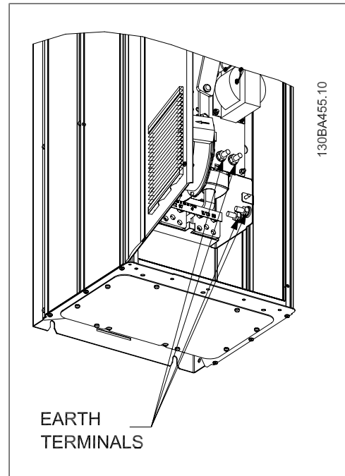
圖 3.75: 地線端子 IP21 (NEMA 類型 1) 與 IP54 (NEMA 類型 12) 的位置
