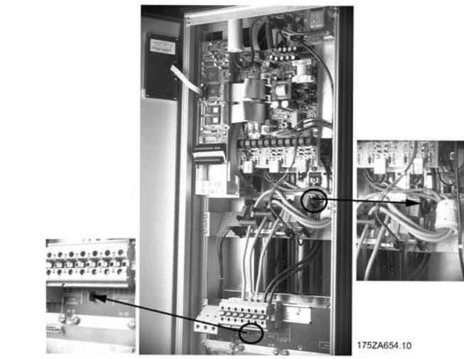
Compact IP 54 VLT 5016-5027 200-240 V VLT 5032-5062 380-500 V
