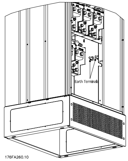
Jordklemmernes positioner, IP 21/IP 54
