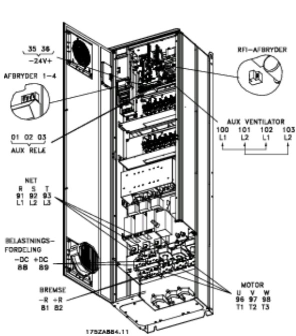
Compact IP 21/IP 54 med afbryder og sikring VLT 5202-5302 380-500 V, VLT 5202-5352 525-690 V Bemærk: RFI-afbryderen har ingen funktion i 525-690 V frekvensomformerne
