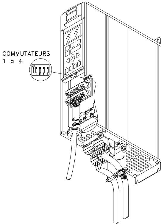
Format livre VLT 5001-5006 200-240 V VLT 5001-5011 380-500 V
