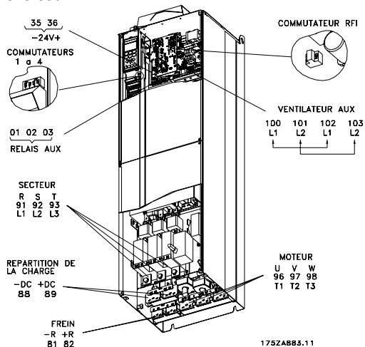
Compact IP21/IP54 avec sectionneur et fusible VLT 5202-5302 380-500 V, VLT 5202-5352 525-690 V
