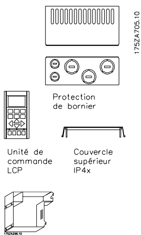
Couvercle inférieur IP 20
