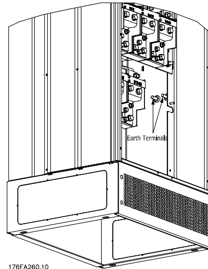
Position des bornes de terre, IP21/IP54
