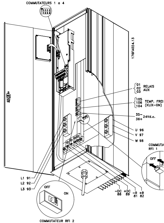
Compact IP54 VLT 5032-5052 200-240 V
