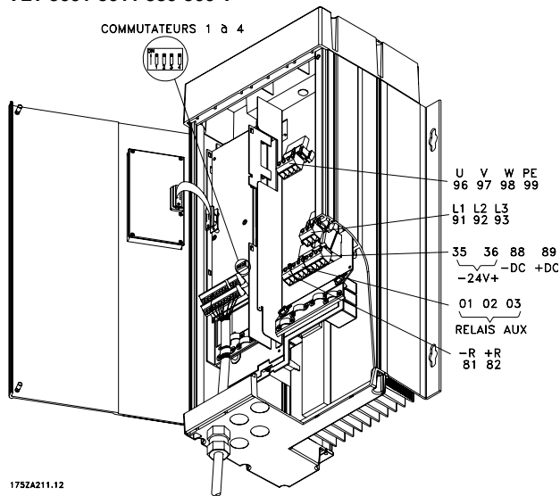
Format livre VLT 5001-5006 200-240 V VLT 5001-5011 380-500 V
