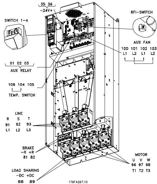
Compact IP 00 sin sistema de desconexión ni fusible VLT 5352-5552 380-500 V, VLT 5402-5602 525-690 V
