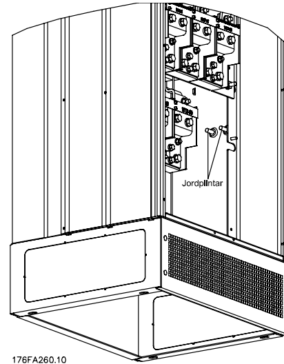
Jordplintarnas position, IP 21/IP 54
