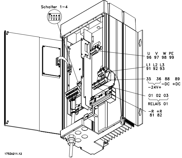
Buchformat VLT 5001-5006 200-240 V VLT 5001-5011 380-500 V
