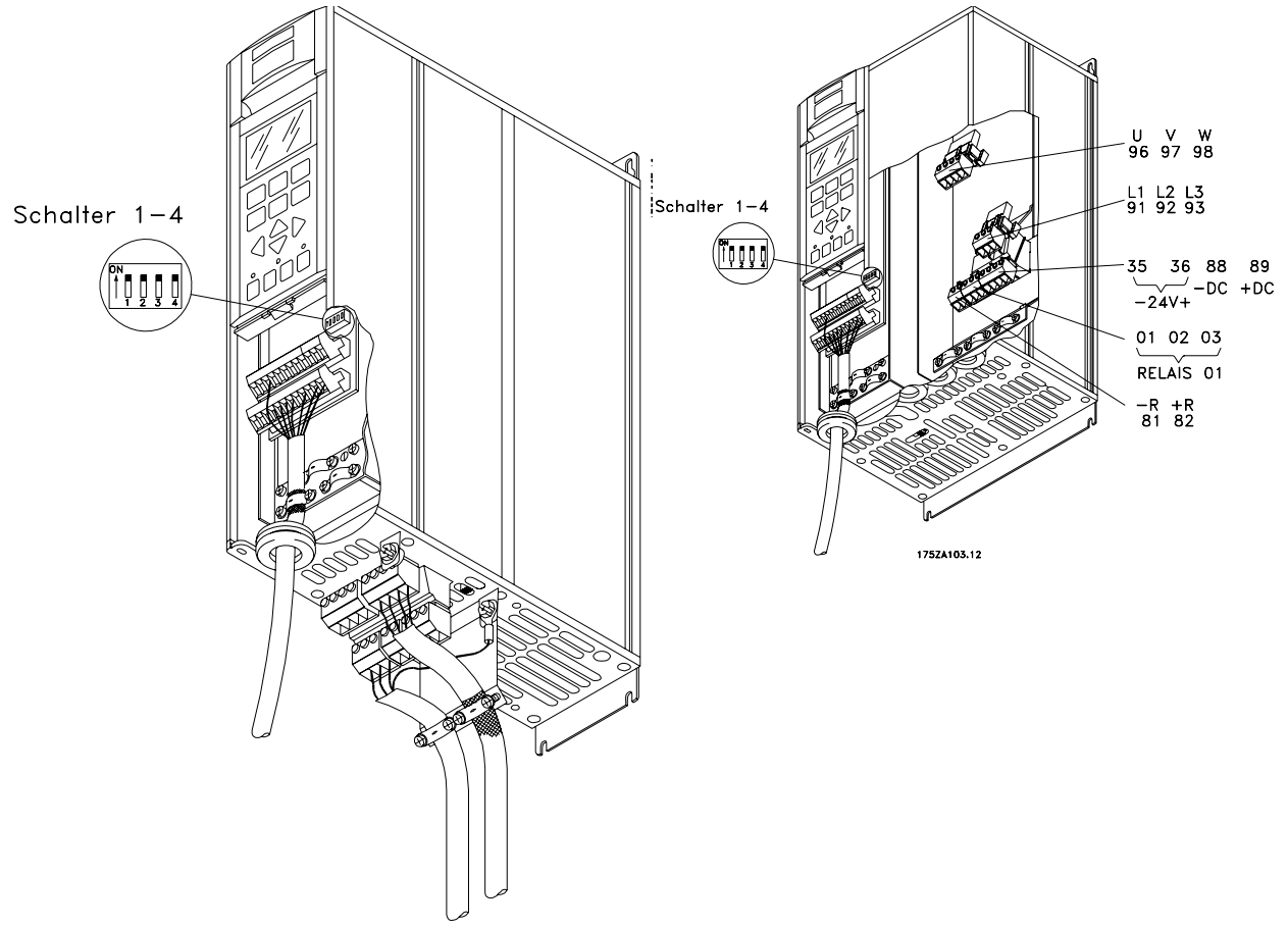
Buchformat VLT 5001-5006 200-240 V VLT 5001-5011 380-500 V
