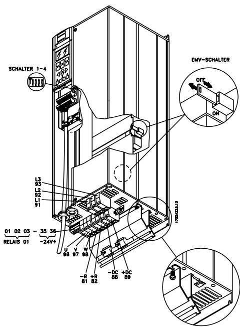
Kompaktformat IP20/NEMA 1 VLT 5008-5027 200-240 V VLT 5016-5062 380-500 V VLT 5016-5062 525-600 V
