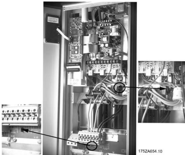
Kompaktformat IP54 VLT 5016 - 5027 200 - 240 V VLT 5032 - 5062 380 - 500 V
