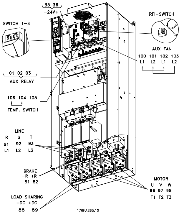
Compact IP 00 med fränkiljare och säkring VLT 5352-5552 380-500 V, VLT 5402-5602 525-690 V
