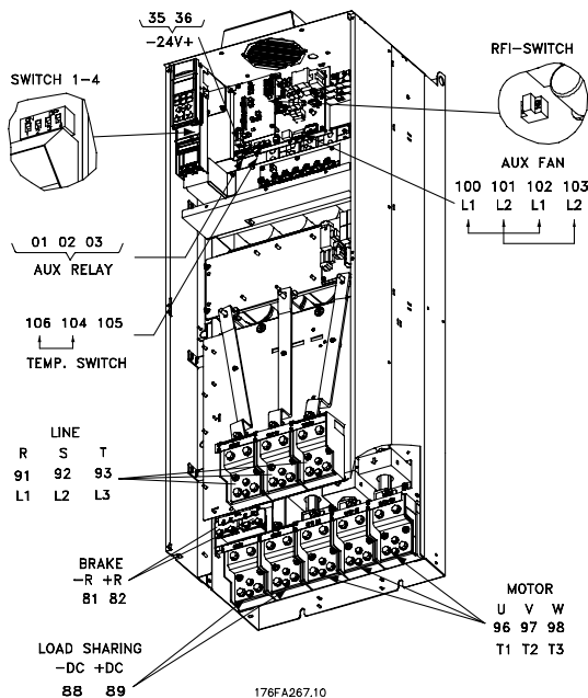
Compact IP 00 utan fränkiljare och säkring VLT 5352-5552 380-500 V, VLT 5402-5602 525-690 V Observera: RFI-switchen fungerar inte i 525-690 V-frekvensomformare.
