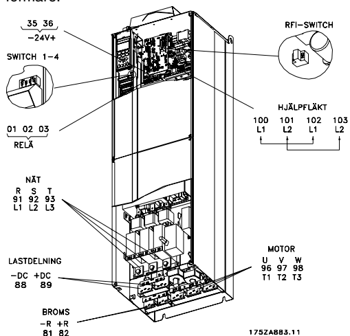
Compact IP 21/IP 54 med fränkiljare och säkring VLT 5202-5302 380-500 V, VLT 5202-5352 525-690 V Observera: RFI-switchen fungerar inte i 525-690 V-frekvensomformare.
