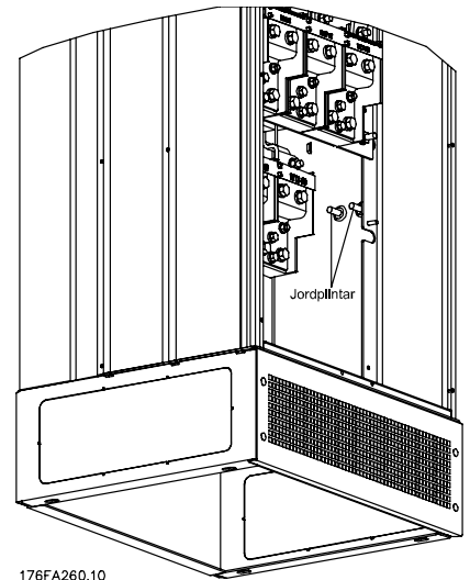
Jordplintarnas position, IP 21/IP 54
