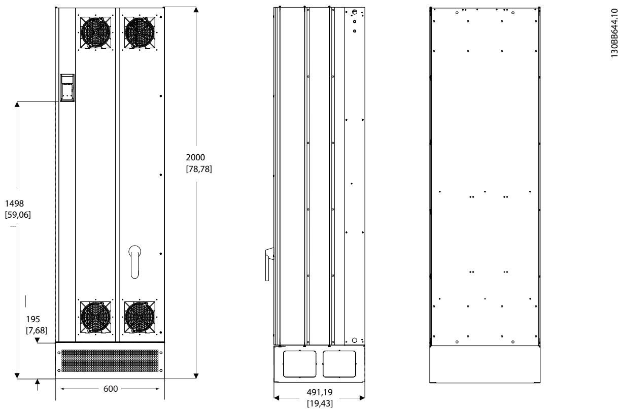
图 4.7 机架规格 E9, AAF06
