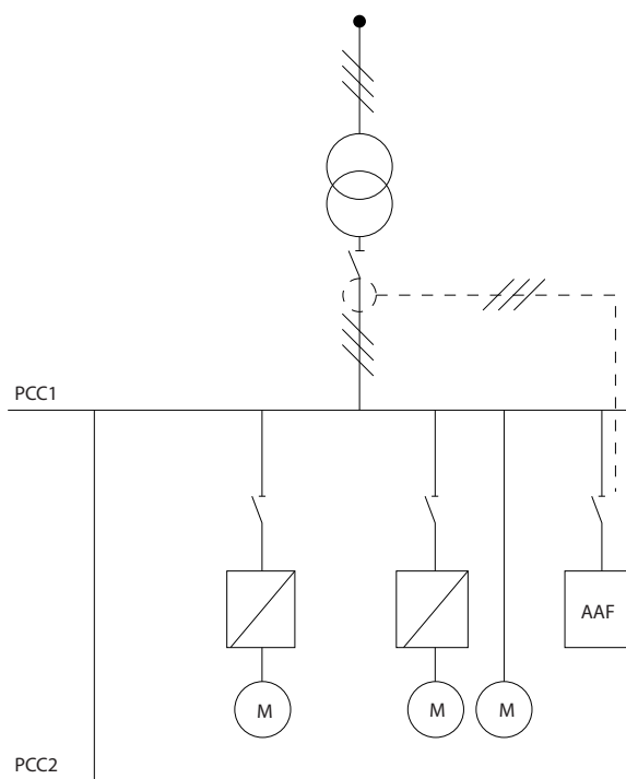
图 4.30 如果变频器安装在整个系统的前部，滤波器将补偿 PCC 侧的变压器 CT 上的所有负载。
