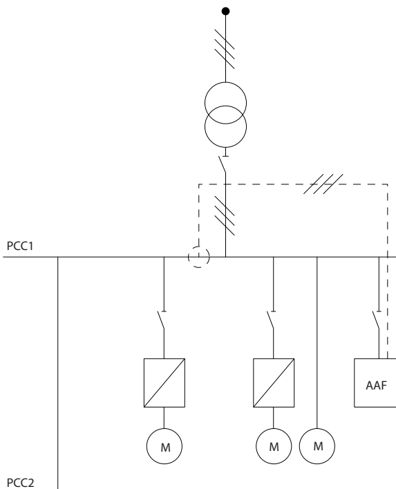
图 4.31 如果变频器安装在配电总线 2 和一台变频器的 前部，滤波器将仅对负载侧的那些 CT 进行电流补偿。
