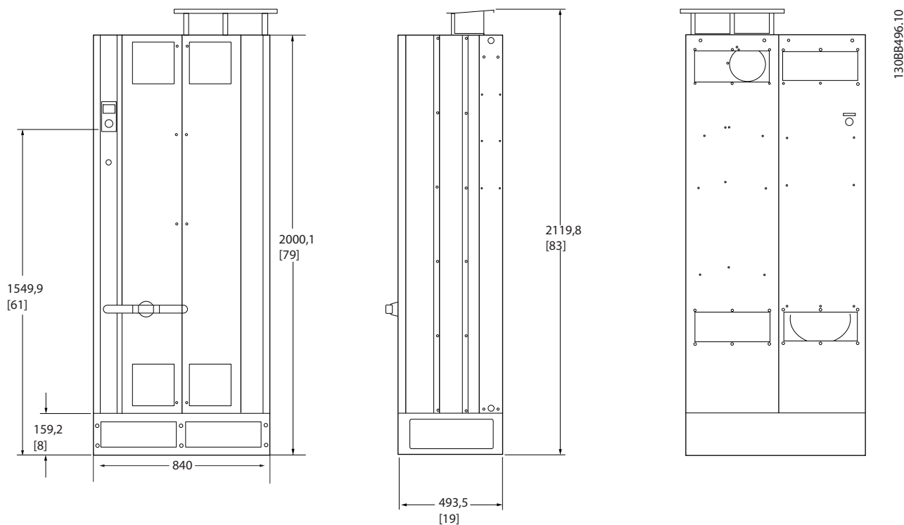
图 4.6 机架规格 E7, AAF05
