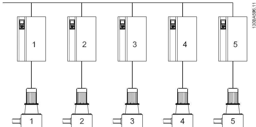
Slika 2.1: Kaskadna kontrola više pumpi
