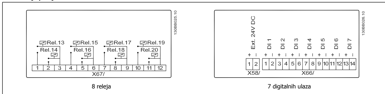
Tablica 2.1: Priključci na naprednom kaskadnom regulatoru MCO 102
