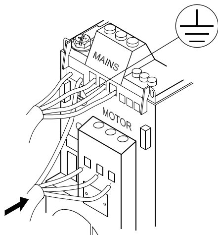
图 1.2 安装接地电缆以及主电源和电机电缆
