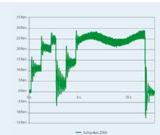
Bei Geräten mit schlankem Zwischenkreis steigt die Neigung zum „Schwingen“ bei größeren Lastwechseln
