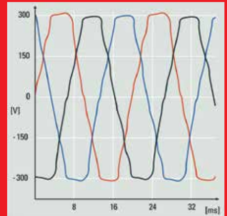
Oscylogram przedstawia wyraźne zniekształcenie napięcia sieci zasilającej spowodowane zakłóceniami pochodzącymi od obciążań o charakterze nieliniowym
