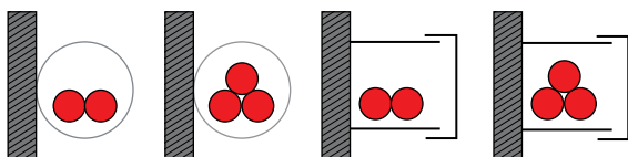
Metoda instalacji B1: Żyły przewodzące w kanałach kablowych, bądź zamknięte w korytkach.
