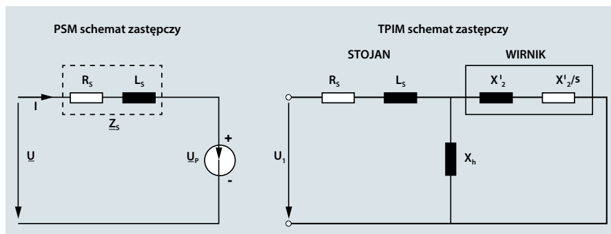
Porównanie schematów zastępczych silników PMSM i TPIM pokazuje brak start w wirniku w silnikach PM/EC. Dzięki temu mają one wyższą sprawność, niż silniki trójfazowe indukcyjne.
