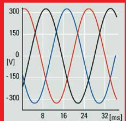
Idealna sytuacja, gdy mamy do czynienia z sinusoidalnym kształtem napięcia zasilającego jest obecnie rzadko spotykana w naszych sieciach energetycznych.
