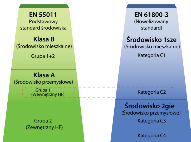
Porównanie nowych kategorii C1 do C4 zdefiniowanych w standardzie produktowym EN 61800-3, oraz klas A i B w standardzie zastosowań EN 55011.
