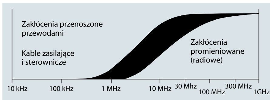
Zakłócenia elektromagnetyczne występują w całym zakresie częstotliwości, jednak ścieżki propagacji oraz forma rozprzestrzeniania są różne.
