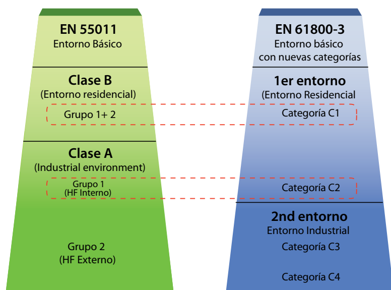
La comparación de las nuevas categorías C1 a C4 definida por la norma de productos EN 61800-3 y las clases A y B de la norma medioambiental EN 55011.
