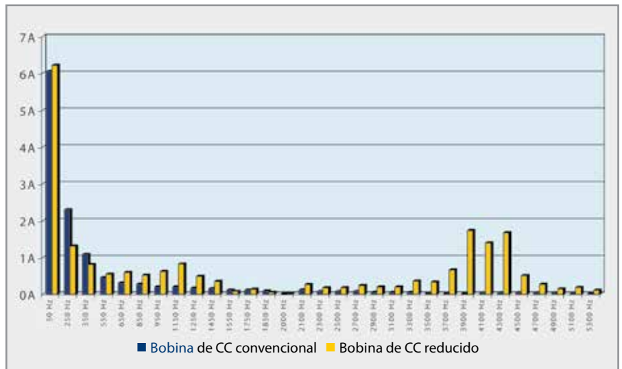
Los convertidores con bobinas de CC reducidos generan niveles armónicos más altos, especialmente en los intervalos de frecuencia más elevados.
