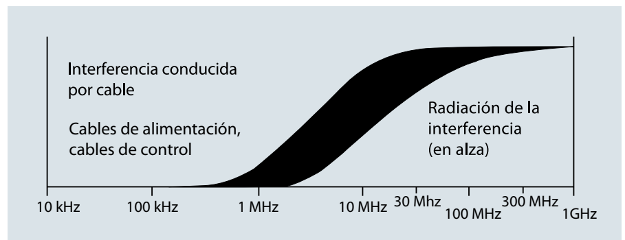
La interferencia electromagnética tiene lugar en todo el rango de frecuencias, pero los trayectos de propagación y la forma de difusión pueden variar.
