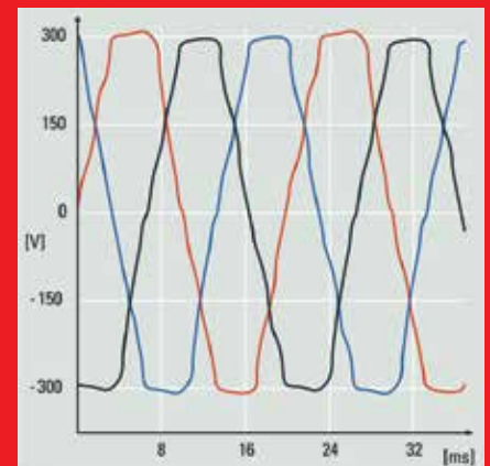
Los cálculos muestran una clara distorsión de la forma de onda de la tensión de red debido a la interferencia de cargas no lineales.
