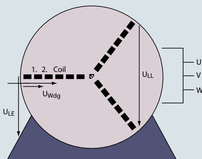
Aparecen tensiones de pulso en el motor en los terminales del motor ( U_{LL} ) y entre los devanados y las láminas ( U_{LE} ). También hay una tensión entre los devanados ( U_{wdg} ).
