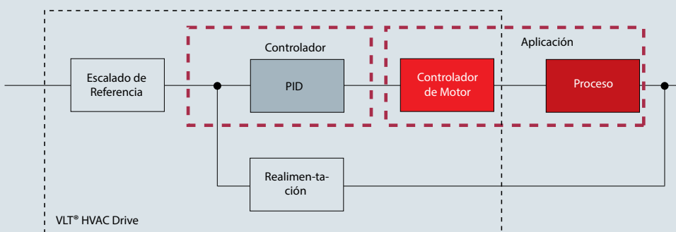
Diagrama de bloques del controlador de proceso PID
