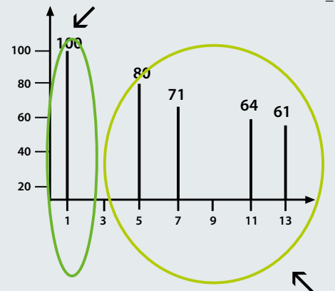
Stromaufnahme des B6 Gleichrichters D
