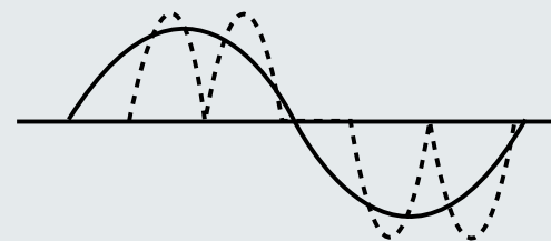
Stromaufnahme des B6 Gleichrichters P
