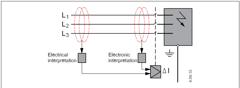
Fig. 6.8 Universal RCCB
