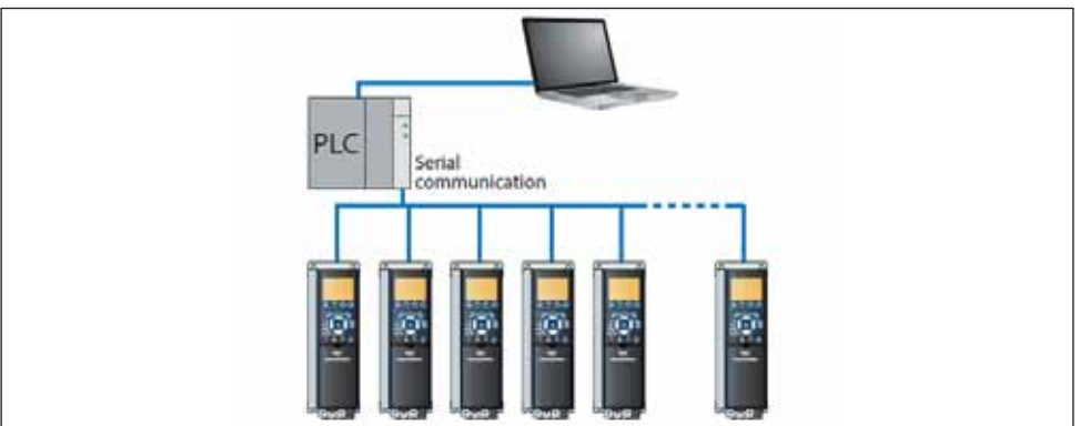
Fig. 8.8 Fieldbus wiring
