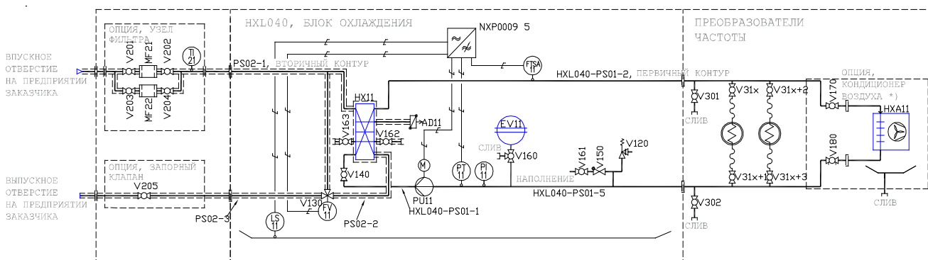
Рисунок 2.2-2. Схема размещения трубопроводов и контрольно-измерительной аппаратуры (КИП)
