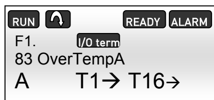
Рисунок 5.1–2. Аварийный сигнал о повышении температуры на панели NXP
