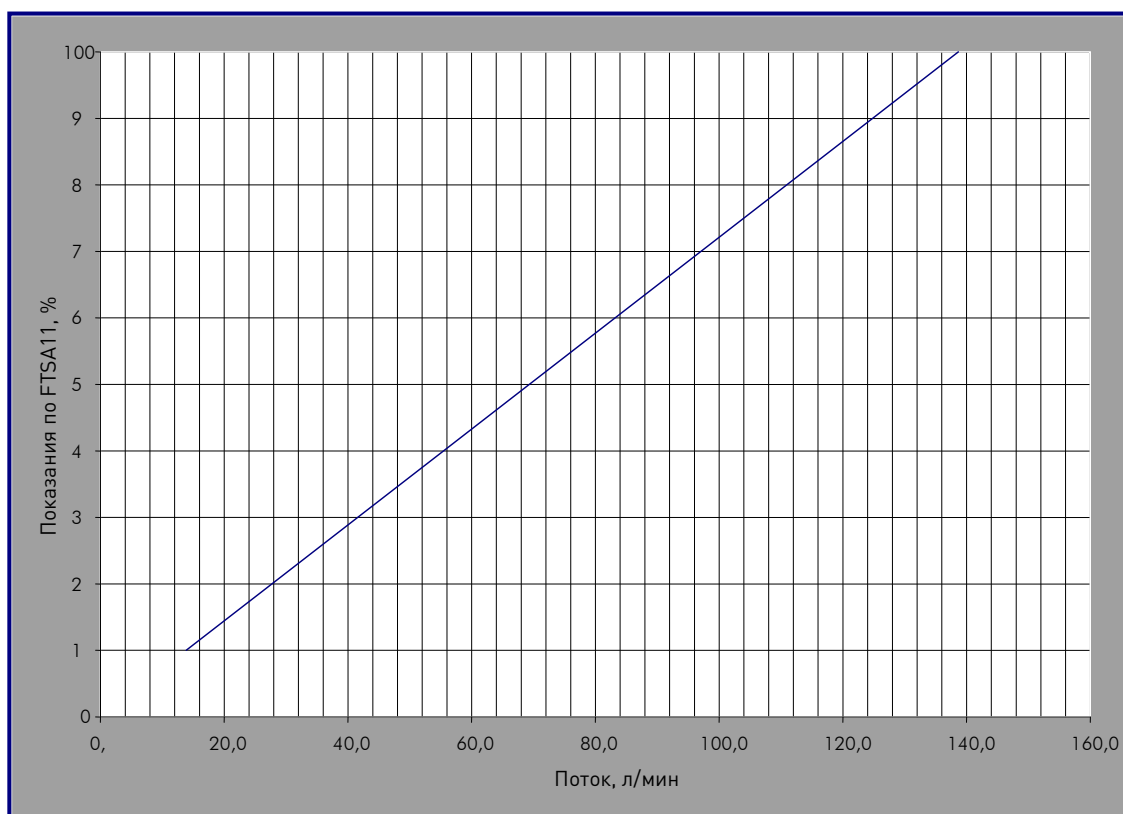
Схема 3.4-1. Переводная таблица реле потока FTSA11 (PVC-C)
