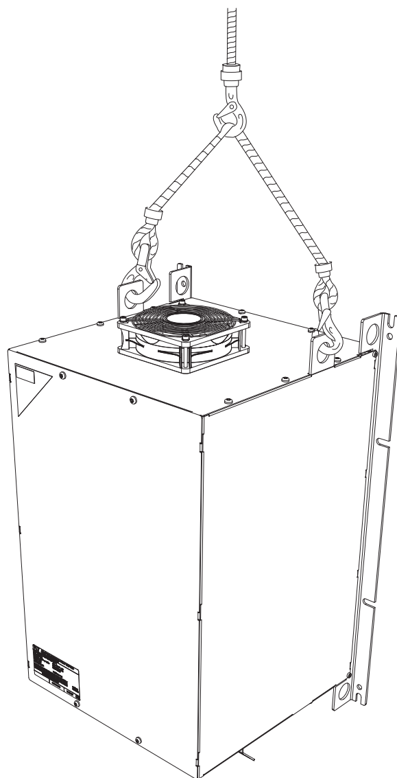
Рисунок 4.2 Рекомендуемый метод подъема, фильтры с внешним вентилятором
