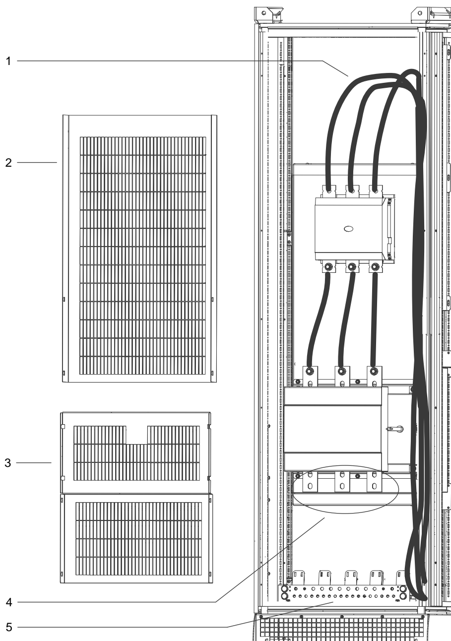
Illustration 50: Points de connexion du secteur à l'option de puissance d'entrée (variateur en armoire configuré sans armoire d'options de puissance)
