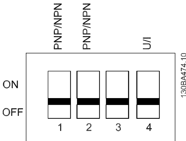
图 1.4 S200 开关 1-4
