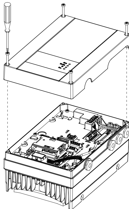
Afbeelding 4.7 Frontafdekking verwijderen
