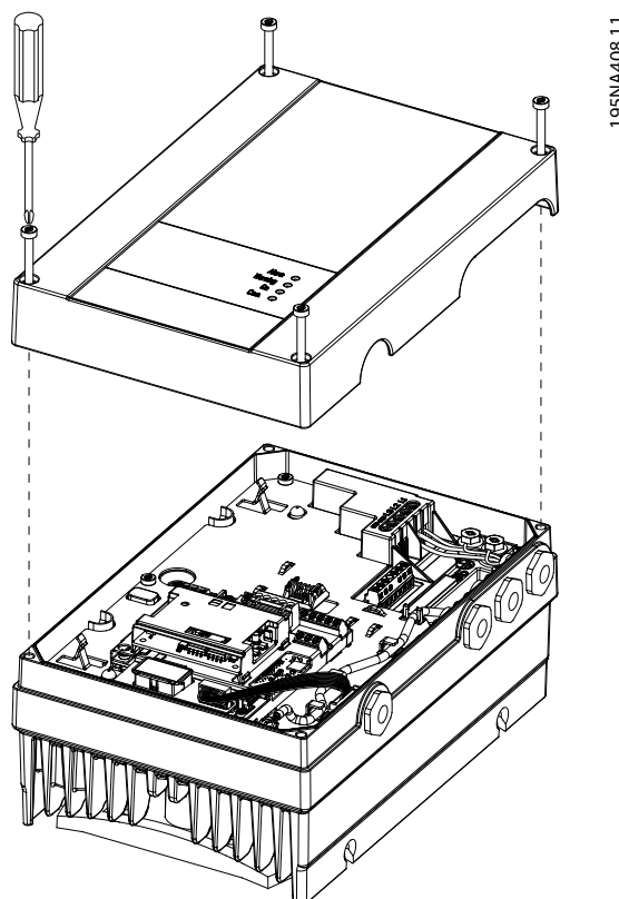
Obrázek 4.7 Sejmutí předního krytu
