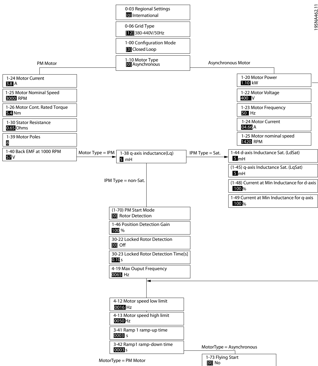
Obrázek 5.9 Nastavení motoru pomocí Rychlého menu
