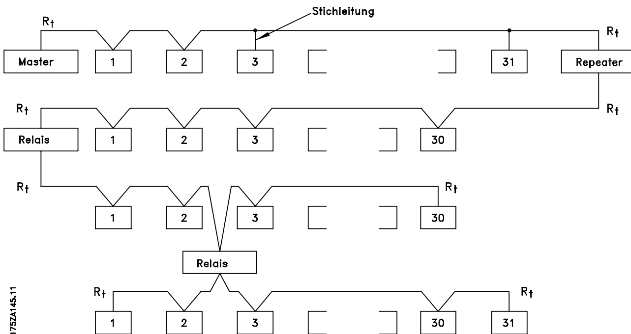
Abbildung 3.1 RS-485-Busschnittstelle
