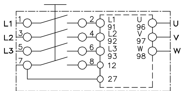
Illustration 4.11 Motor- og nettilslutning med servicekontakt
