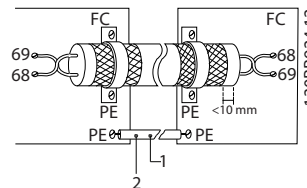
图 3.10 双绞电缆（无端子 61）
