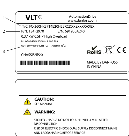
图 1.1 铭牌 1 和 2
