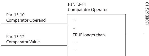
Рисунок 2.36 Компараторы
