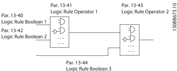
Рисунок 2.37 Правила логики
