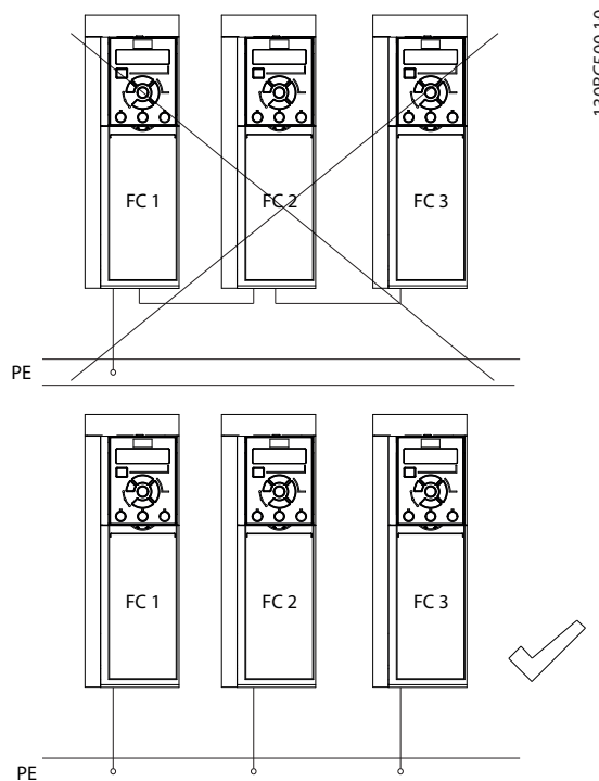
图 2.3 接地原理
