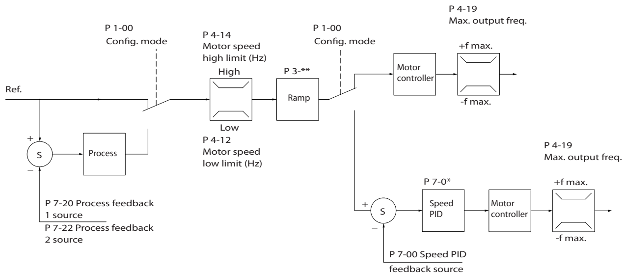
图 2.14 VVC+ 开环和闭环配置下的控制结构
