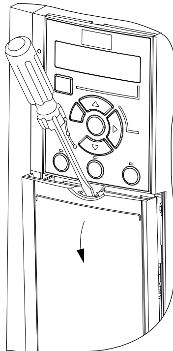
图 2.6 J1-J7 机箱规格的控制线路检视
