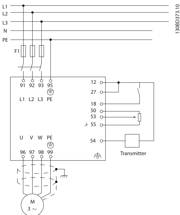
图 2.27 2 线传感器
