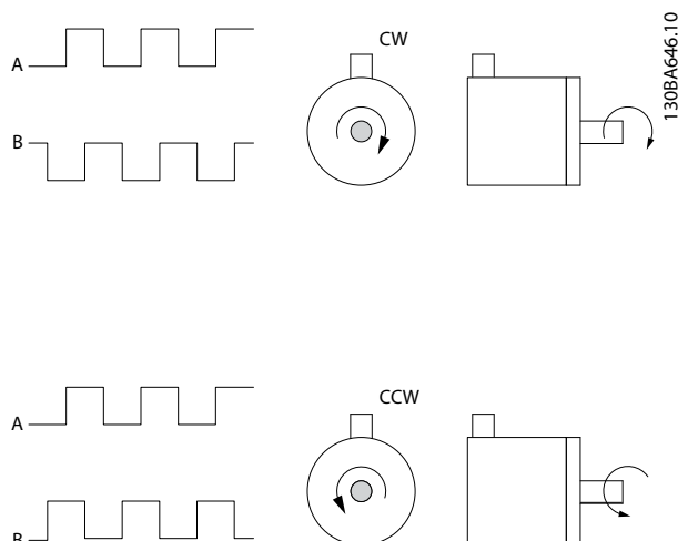
图 6.3 24 V 增量型编码器, 最大电缆长度 5 米 (16.4 英尺)
