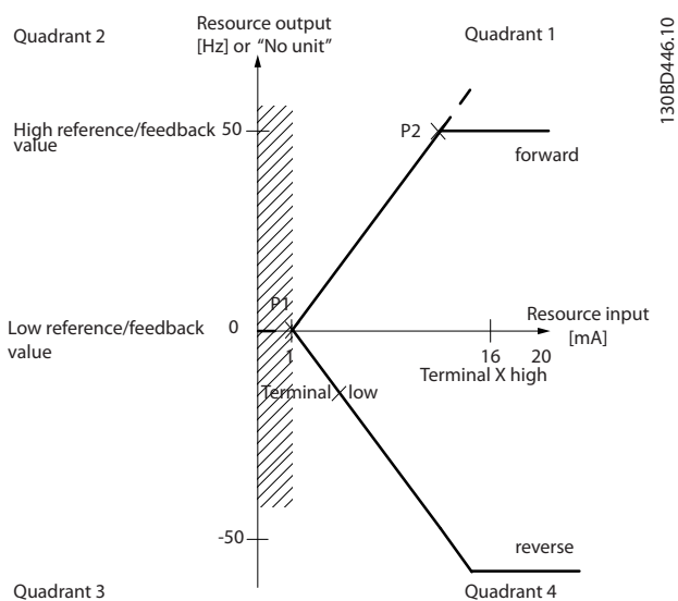
图 2.21 死区大小
