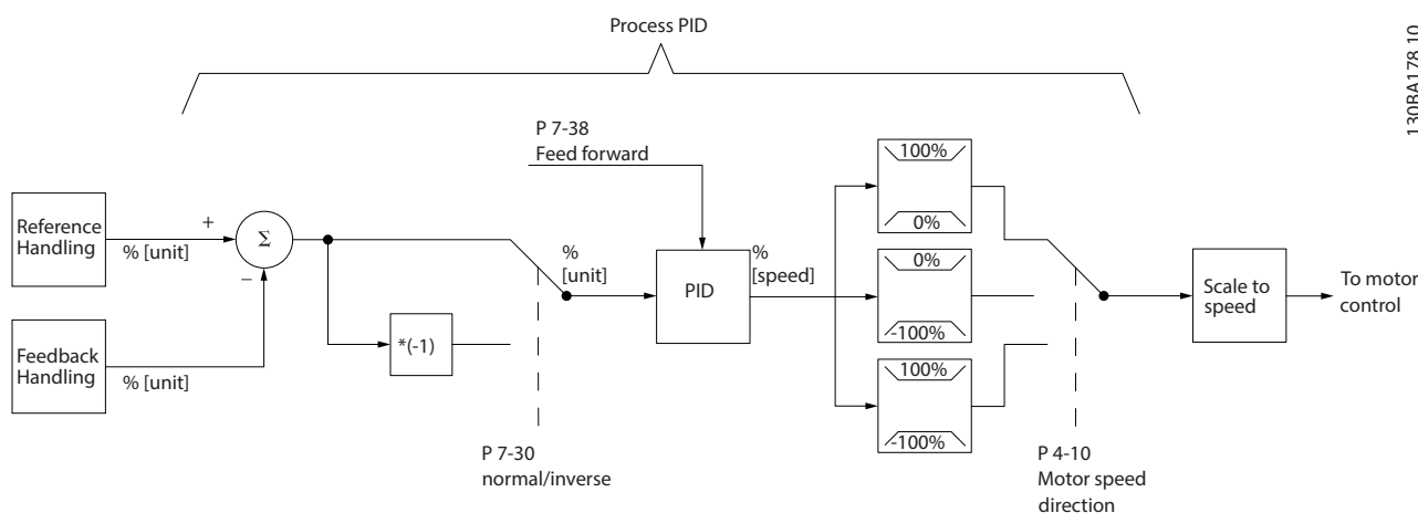
图 2.25 过程 PID 控制图
