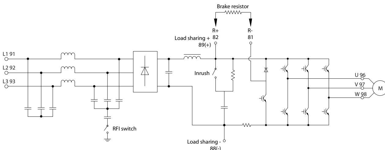
图 2.12 FC 360 0.37 - 22 kW (0.5 - 30 hp) 的控制图
