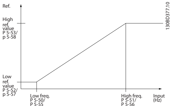
图 4.13 脉冲输入
