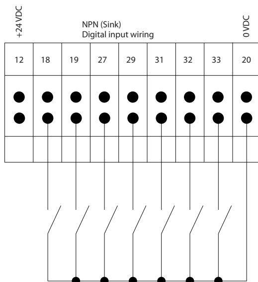
图 1.5 NPN (漏型)
