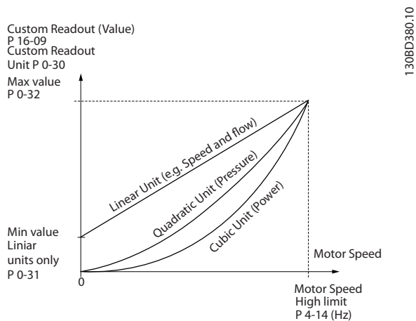
图 4.1 自定义读数
