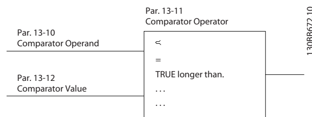
图 4.23 比较器
