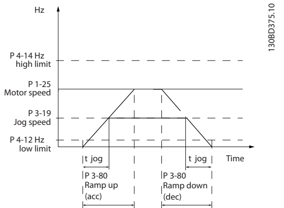
图 4.8 点动加斜坡时间
