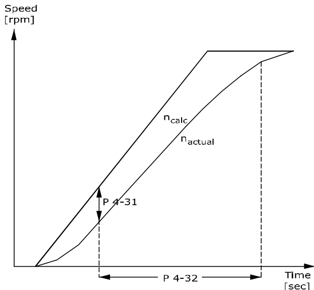
图 4.10 电机反馈速度错误
