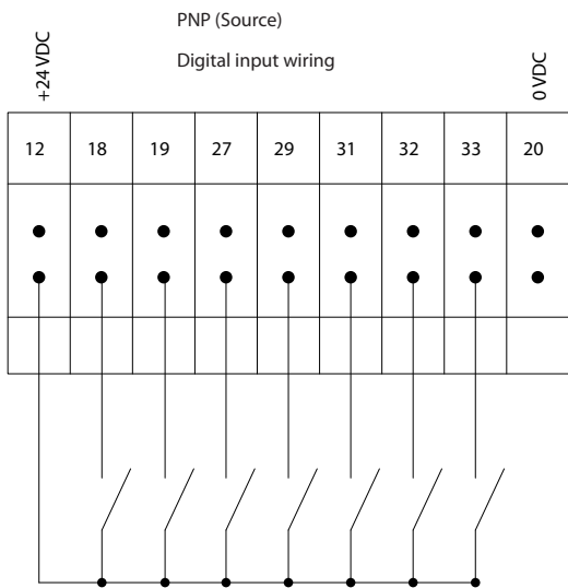
图 1.4 PNP (源型)
