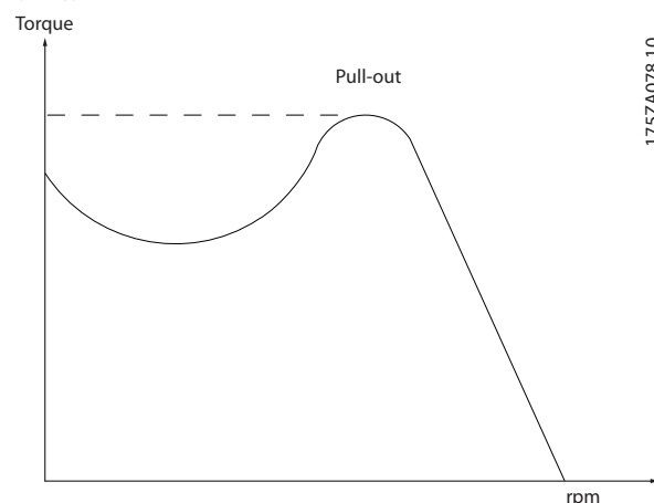
图 1.2 起步转矩
