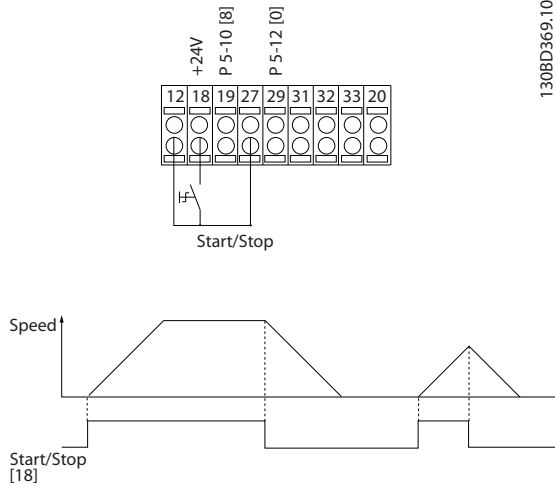
图 1.7 启动/停止
