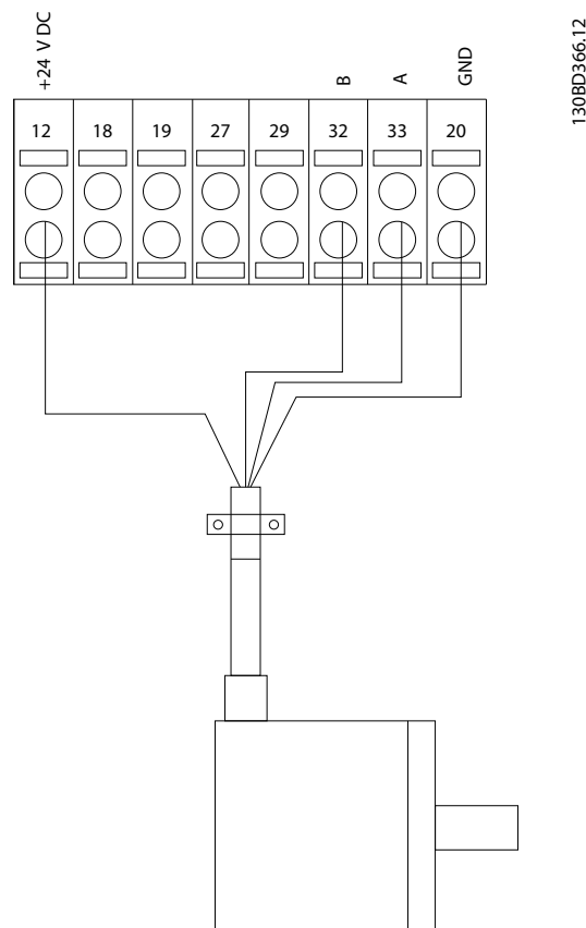
图 4.15 24 V 或 10-30 V 编码器连接
