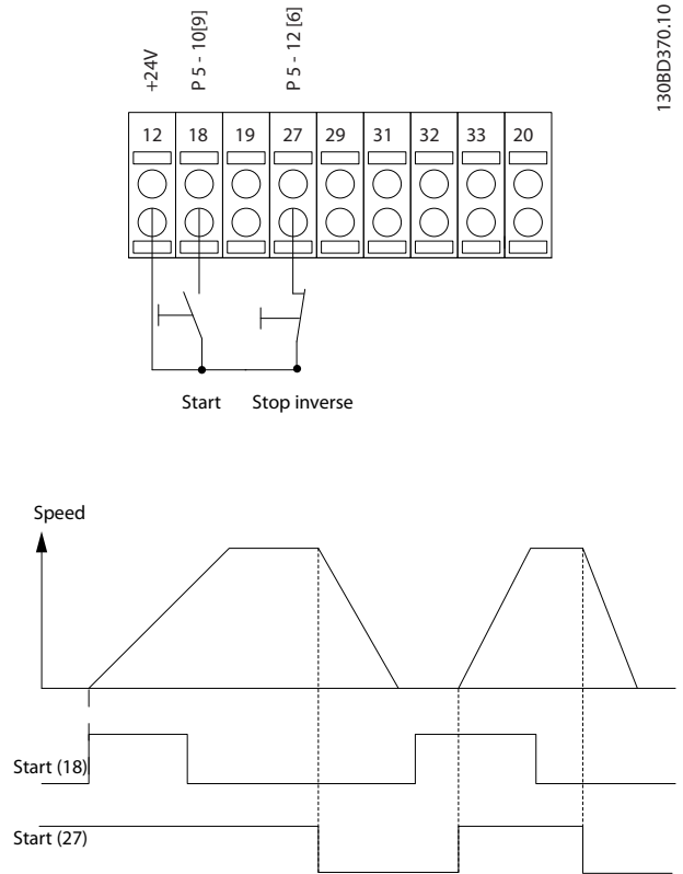
图 1.8 脉冲启动/停止
