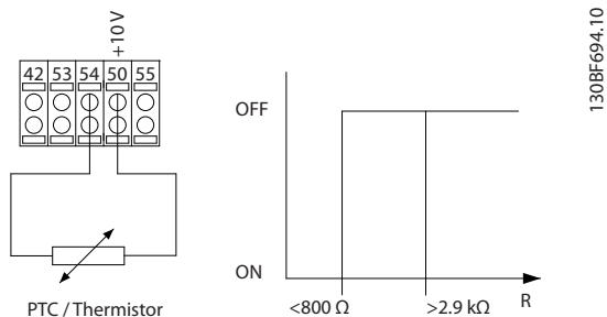
Ilustração 4.6 Conexão do termistor PTC - Entrada analógica
