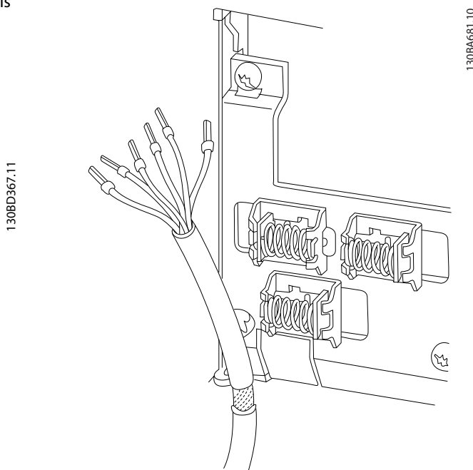
Ilustração 1.5 Aterramento de cabos de controle blindados/reforçados
