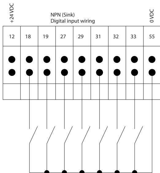
Ilustração 1.4 NPN (Dissipador)
