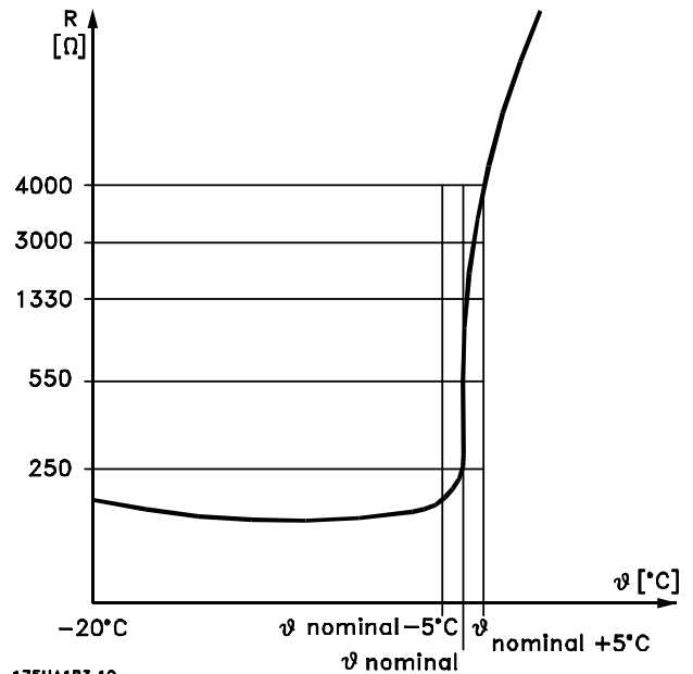
175HA183.10 Ilustração 4.4 Perfil do PTC
