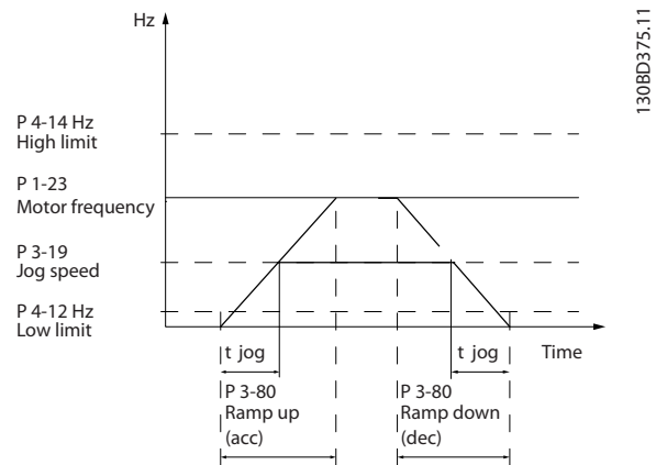
Ilustração 4.11 Tempo de Rampa do Jog
