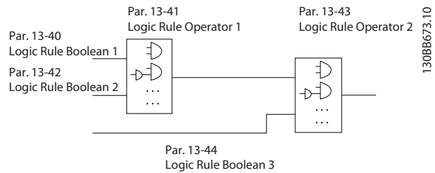
Ilustração 4.28 Regras Lógicas
