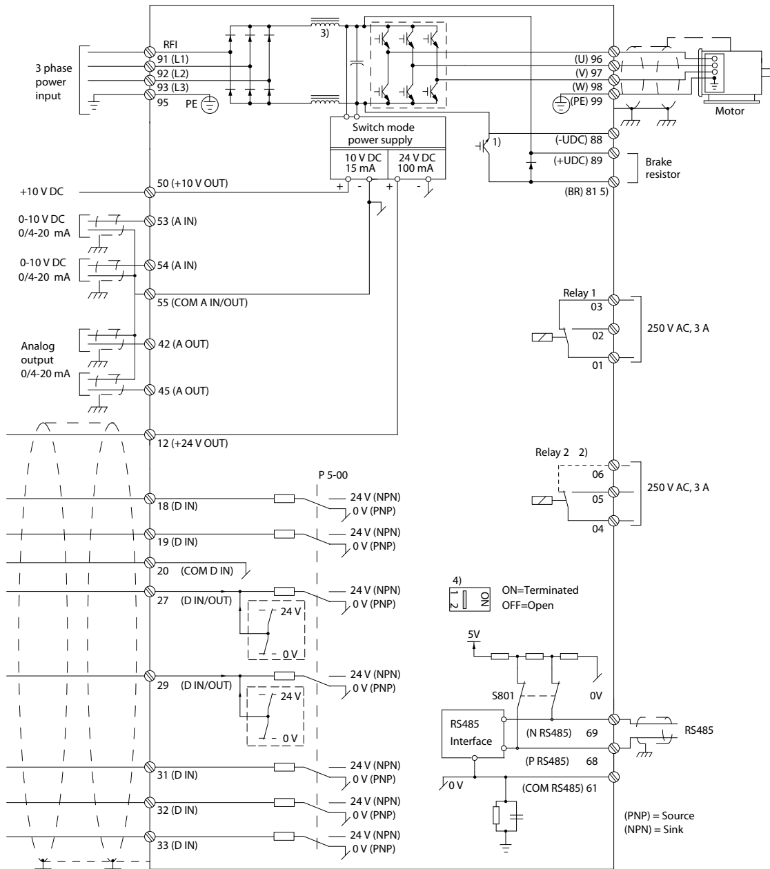
Ilustração 1.2 Diagrama Esquemático de Fiação Básica
