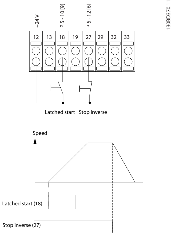
Ilustração 1.7 Partida por pulso/Parada por inércia inversa
