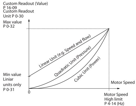
Ilustração 4.1 Leitura Personalizada
