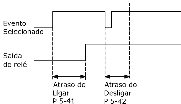
Ilustração 4.16 Atraso de desligamento, relé
