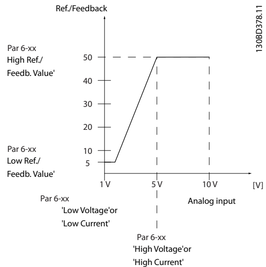
Ilustração 4.21 Função Timeout
