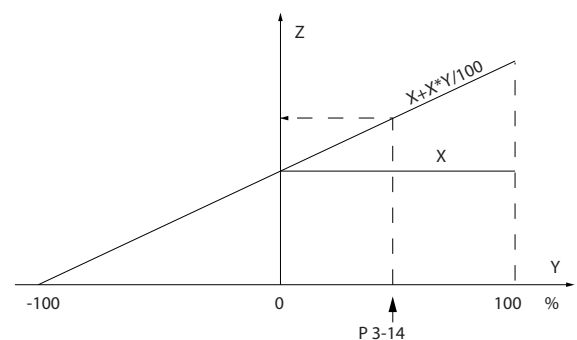
Ilustração 4.8 Referência real
