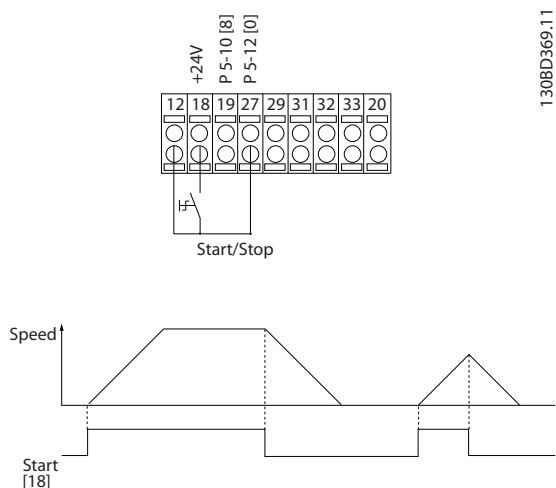
Ilustração 1.6 Partida/Parada
