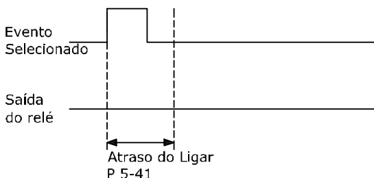
Ilustração 4.15 Atraso de Ativação do Relé
