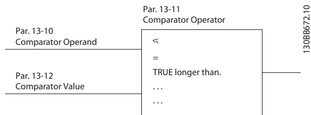
Ilustração 4.27 Comparadores
