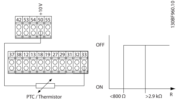
Ilustração 4.5 Conexão do termistor PTC - Entrada digital
