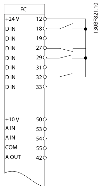
Ilustração 1.8 Aceleração/Desaceleração
