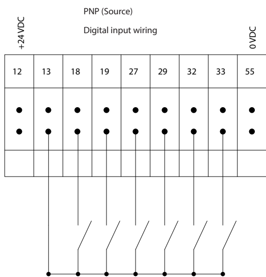
Ilustração 1.3 PNP (Origem)
