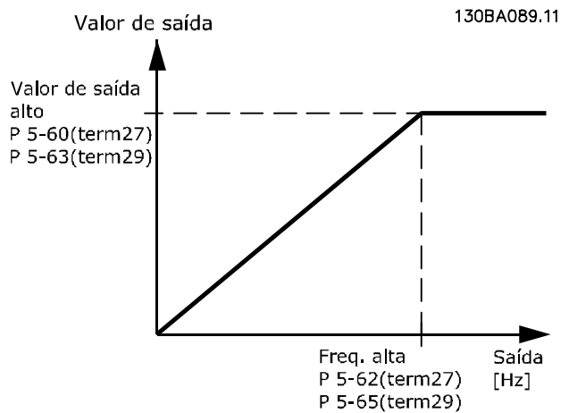
Ilustração 4.18 Configuração das Saídas de Pulso
