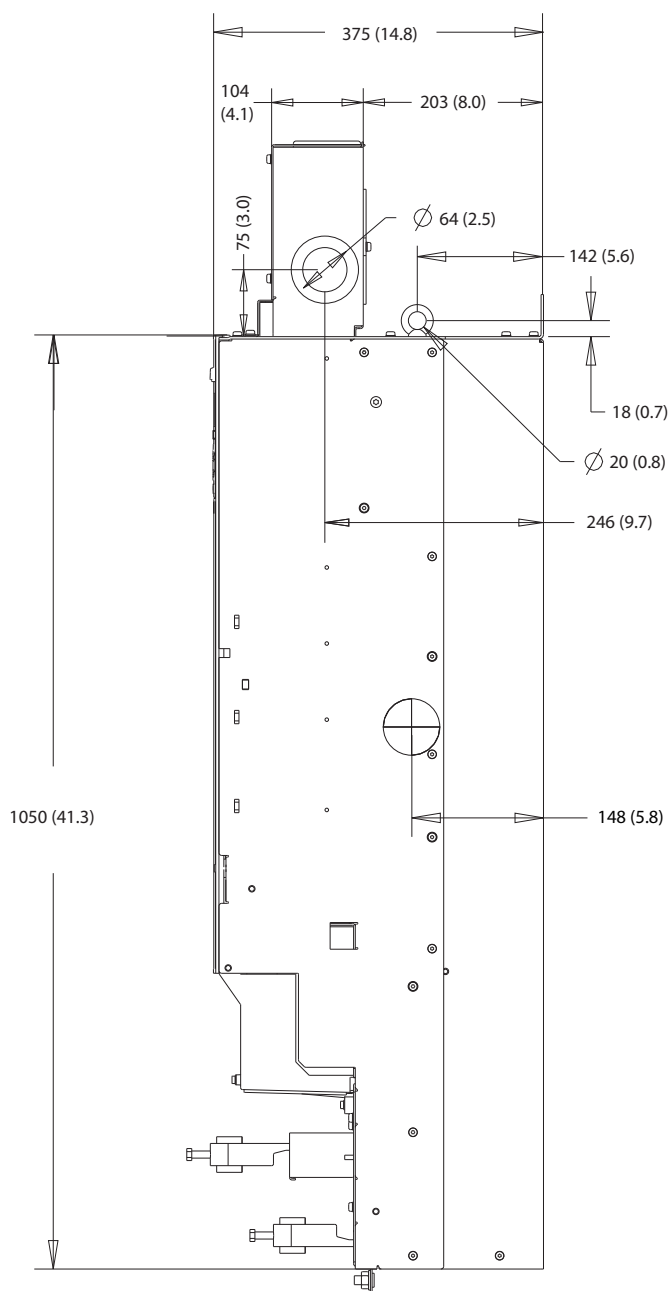
图 10.6 J9 的侧视图
