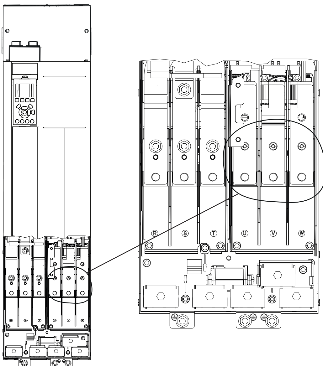
图 5.4 电机端子 (所示为 J8)
