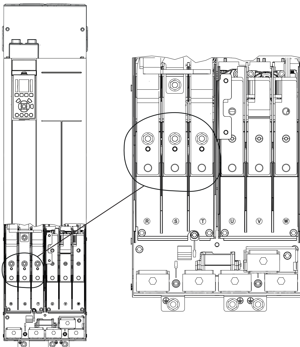
图 5.5 交流主电源端子（所示为 J8）。有关端子的详细视图，请参考章 5.7 端子尺寸。
