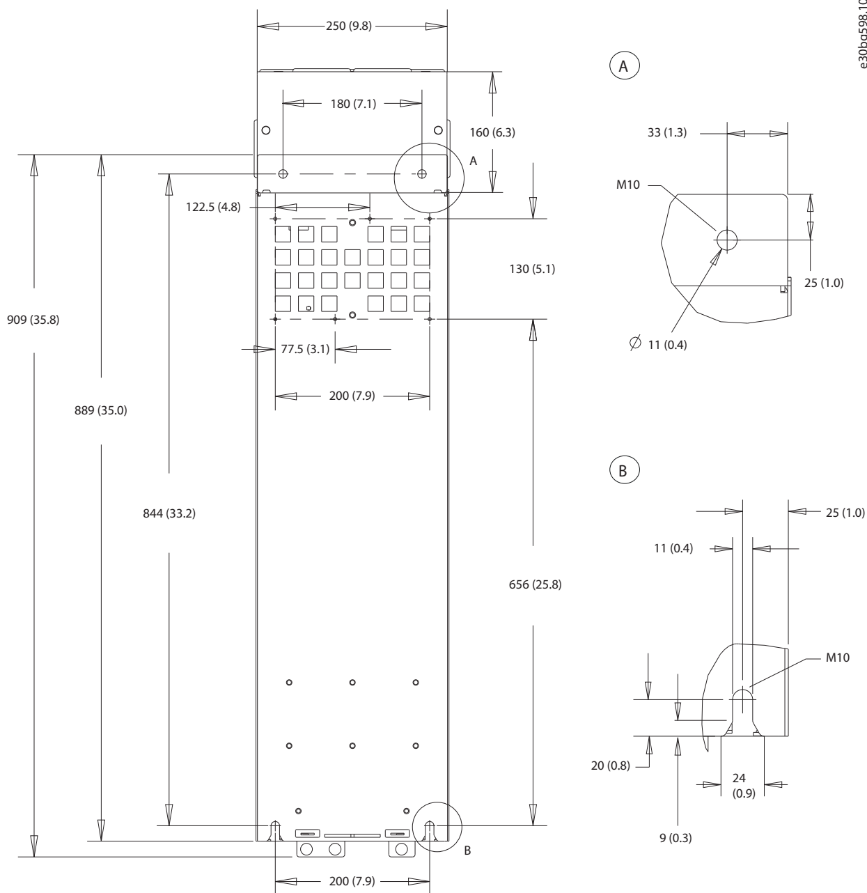
图 10.4 J8 的后视图
