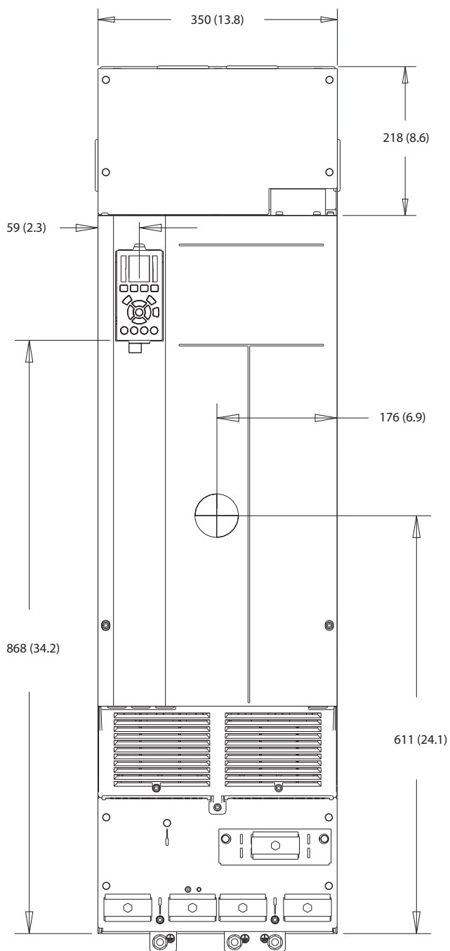
图 10.5 J9 的前视图
