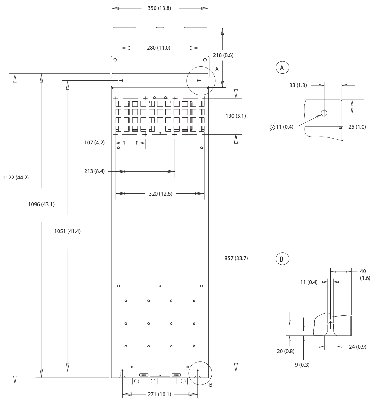
图 10.7 J9 的后视图
