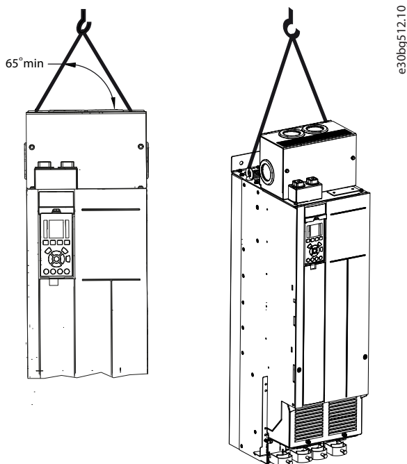
图 4.2 起吊变频器
