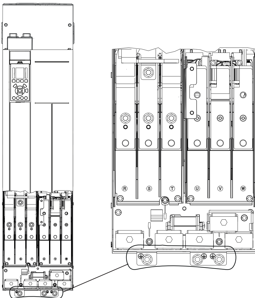
图 5.3 接地端子 (所示为 J8)
