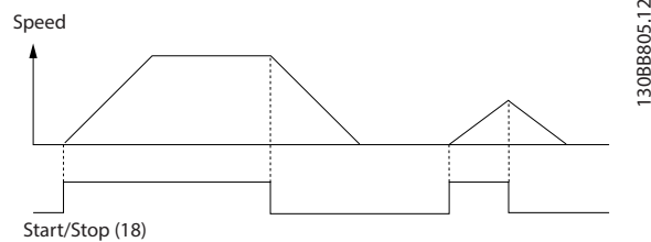
图 8.2 启动/停止命令
