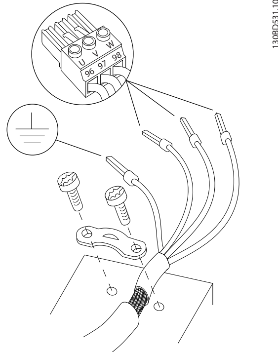
Ábra 4.5 Motorcsatlakoztatás
