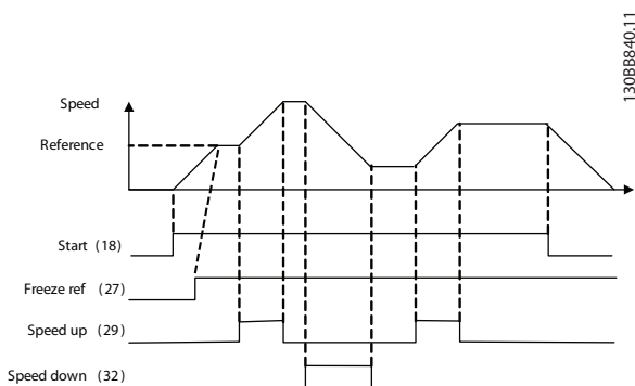
Ábra 7.1 Fordulatszám növelése/csökkentése
