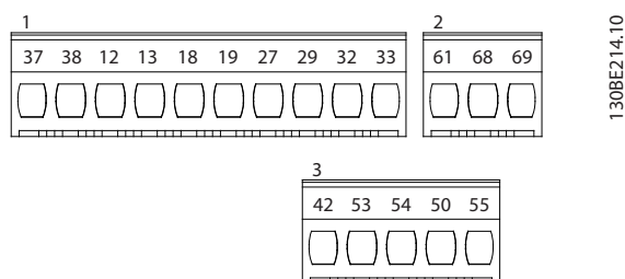
Ábra 4.10 Csatlakozószámok
