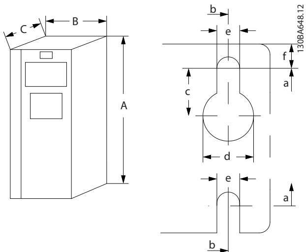
Illustration 9.5 Øverste og nederste monteringshuller
