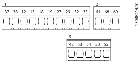
Kuva 4.10 Liitinten numerot
