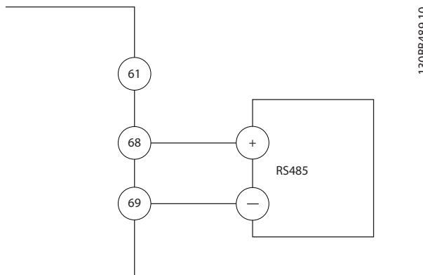
Kuva 4.14 Sarjaliikenteen kytkentäkaavio
