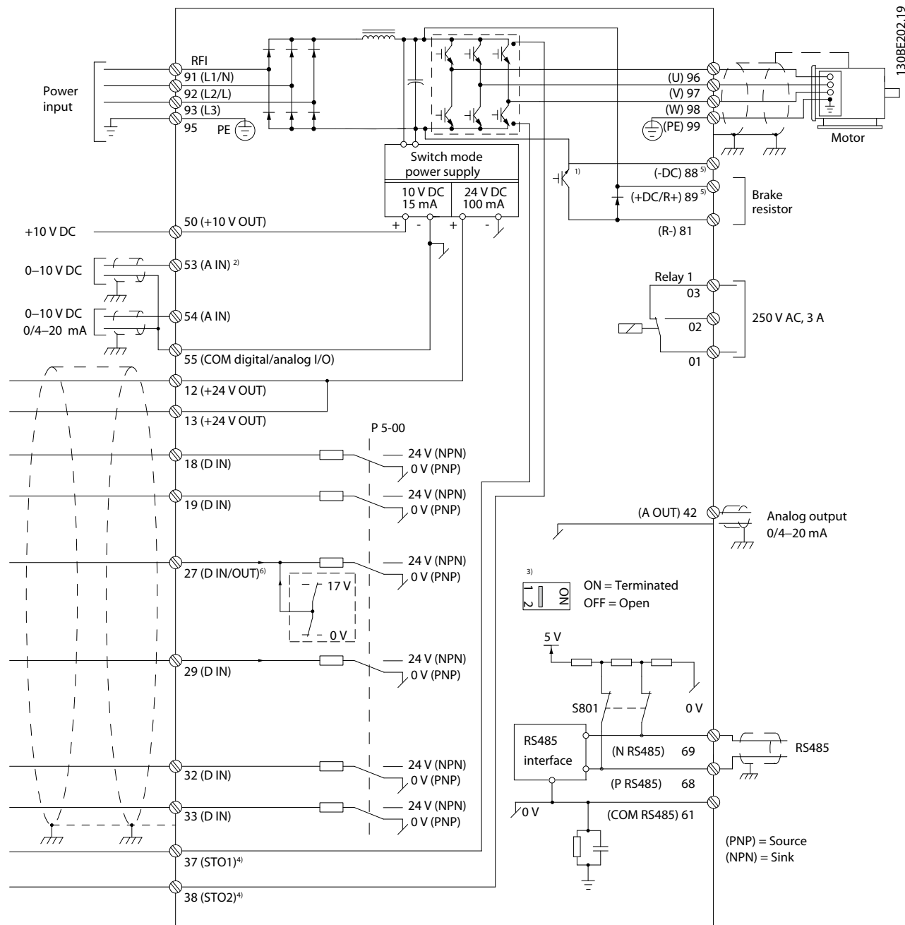
图 4.2 基本接线示意图
