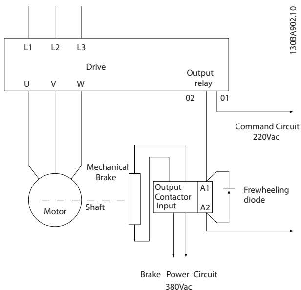
图 2.25 将机械制动连接到 变频器
