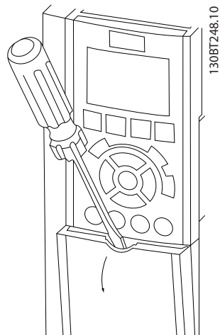
图 2.13 A2、A3、B3、B4、C3 和 C4 机箱的控制端子检视
