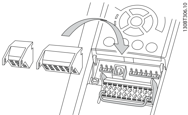
图 2.16 拔下控制端子
