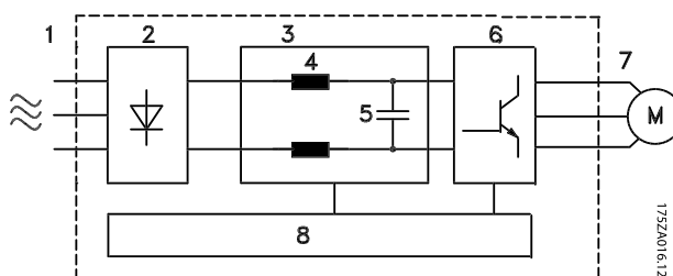
图 1.3 变频器框图
