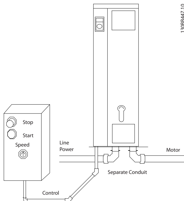
图 2.6 使用线管执行的正确电气安装
