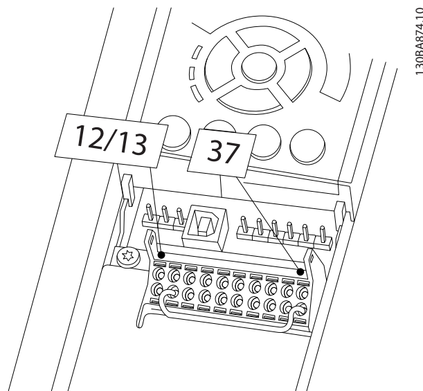
图 2.23 端子 12/13 (24 V) 与 37 之间的跳线
