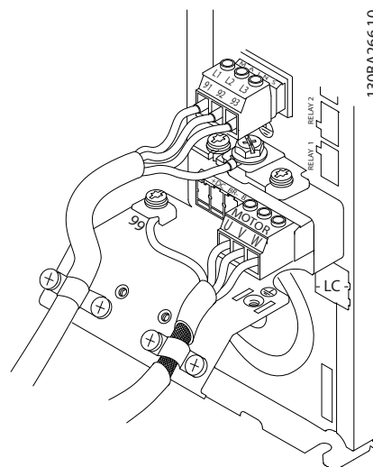
图 2.8 使用屏蔽电缆接地
