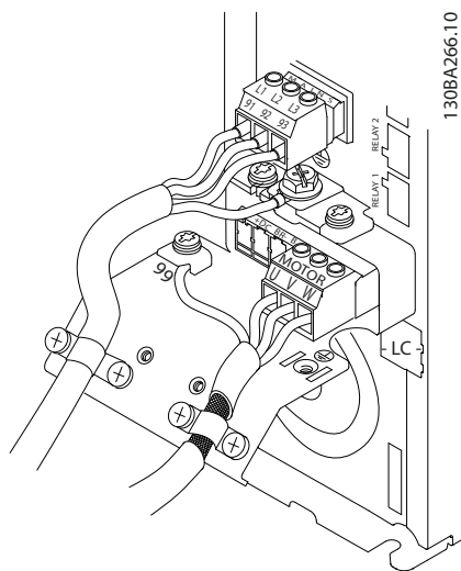
图 2.9 A-机架规格的电动机接线、主电源接线以及接地
