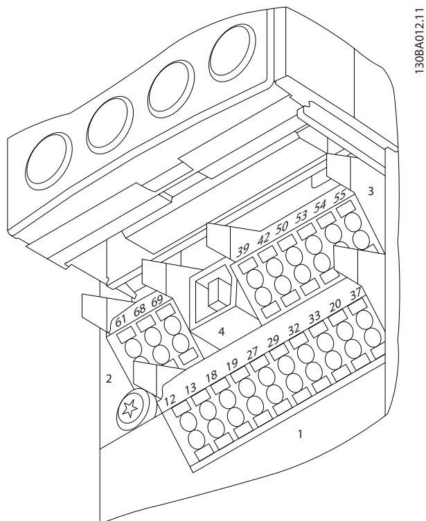
图 2.15 控制端子位置
