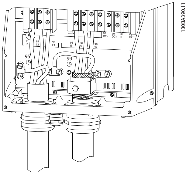
图 2.10 B-机架规格以及之上机架规格的电动机接线、主电源接线以及接地（使用屏蔽电缆）
