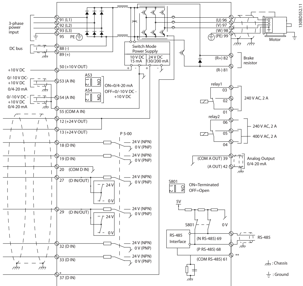
Slika 4.1 Šematski prikaz osnovnog ožičenja
