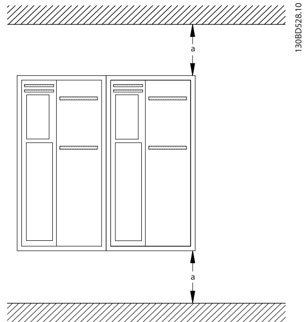
Slika 3.4 Gornji i donji zazor za hlađenje
