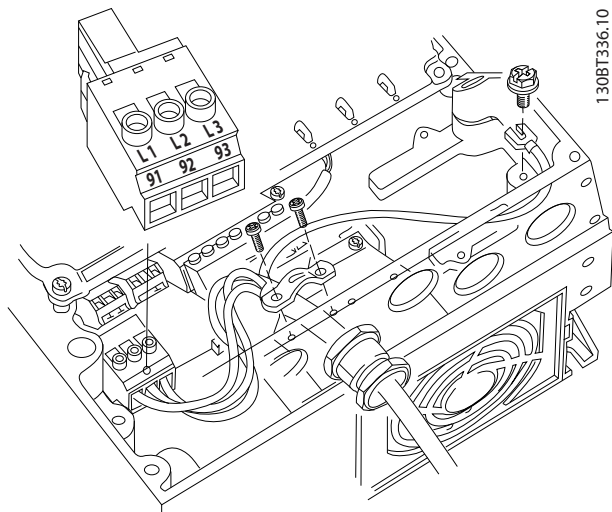
Slika 4.9 Priklučivanje na mrežno napajanje naizmeničnom strujom
