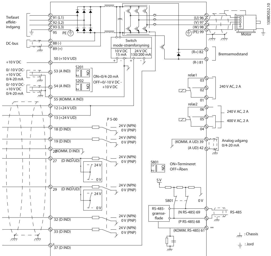
Illustration 4.1 Grundlæggende ledningsdiagram
