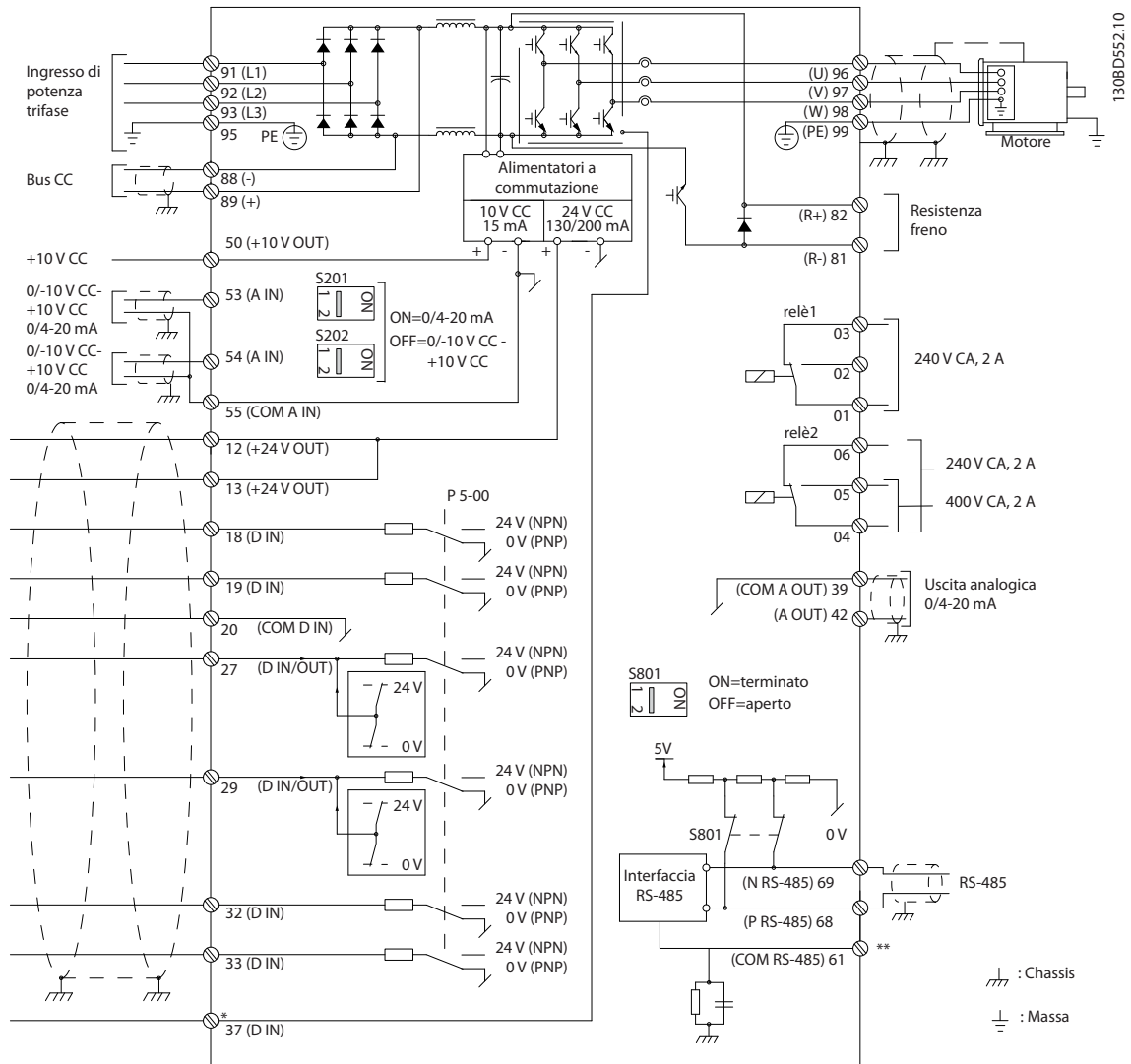
Disegno 4.1 Schema di cablaggio di base
