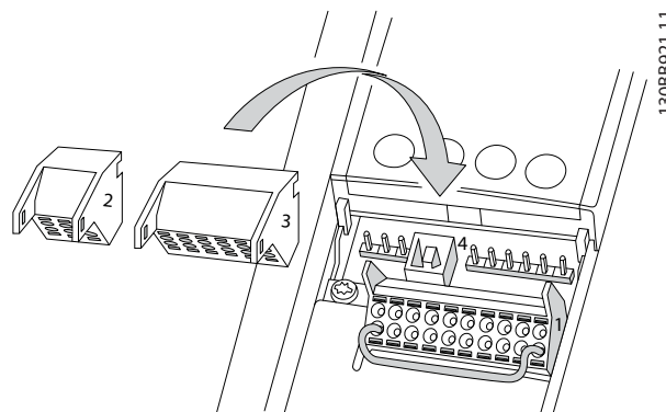
Slika 4.10 Lokacije upravljačkih stezaljki
