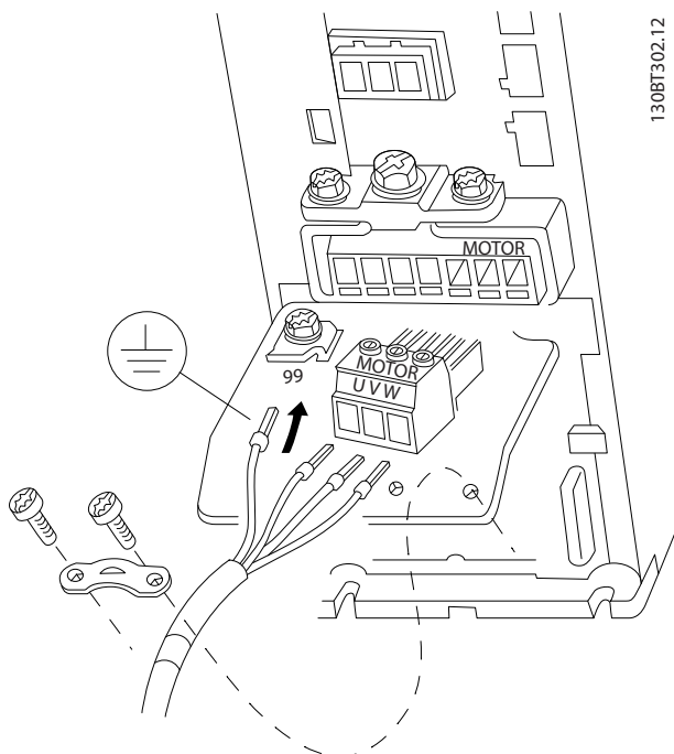
Slika 4.6 Priklučivanje motora za tip kućišta A2 i A3
