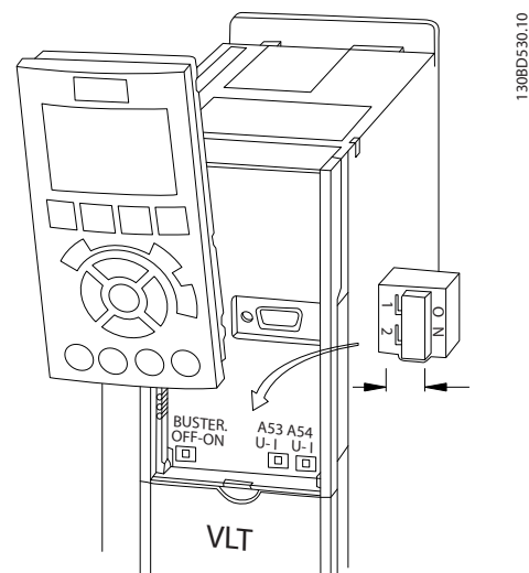
Slika 4.13 Lokacija sklopki stezaljki 53 i 54
