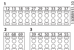
그림 4.11 단자 번호
