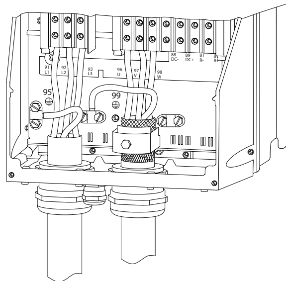
그림 4.8 차폐 케이블을 사용한 외함 유형 B 및 C의 모터, 주전원 및 접지 배선
